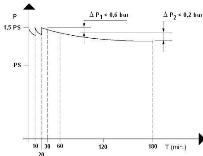
Fig. 1: Procédure du contrôle d'étanchéité
