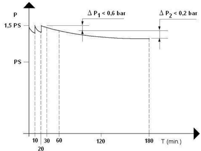
Fig. 1: Procédure du contrôle d'étanchéité
