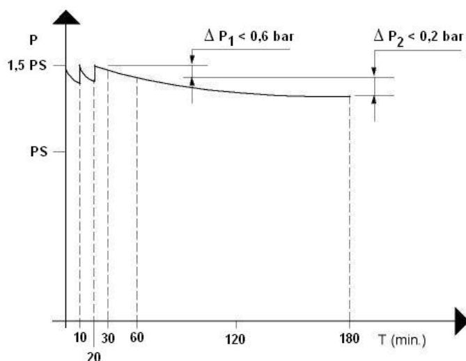
Fig. 1 Procedure dichtheidscontrole
