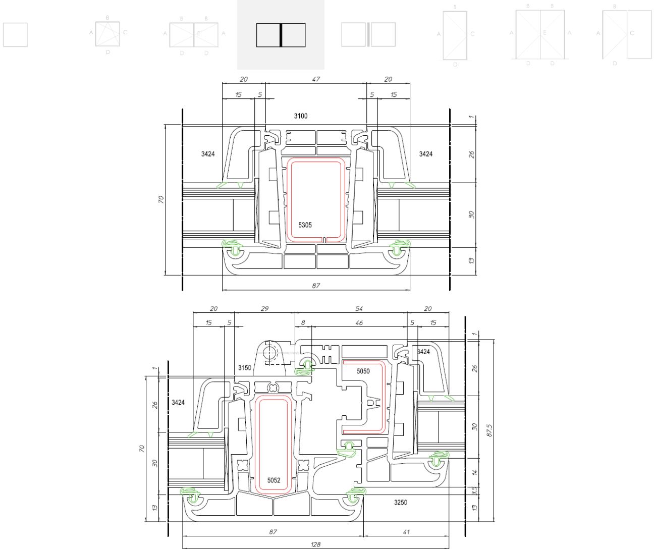
Figuur 9d: Typesnede samengesteld venster
