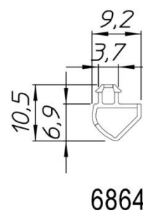
Figuur 6b – Middendichting
