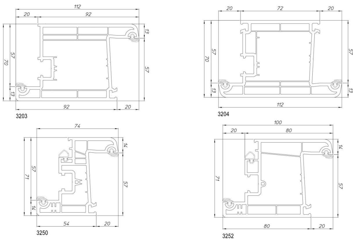
Figuur 2 – Weerstandsp profielen – vleugel
