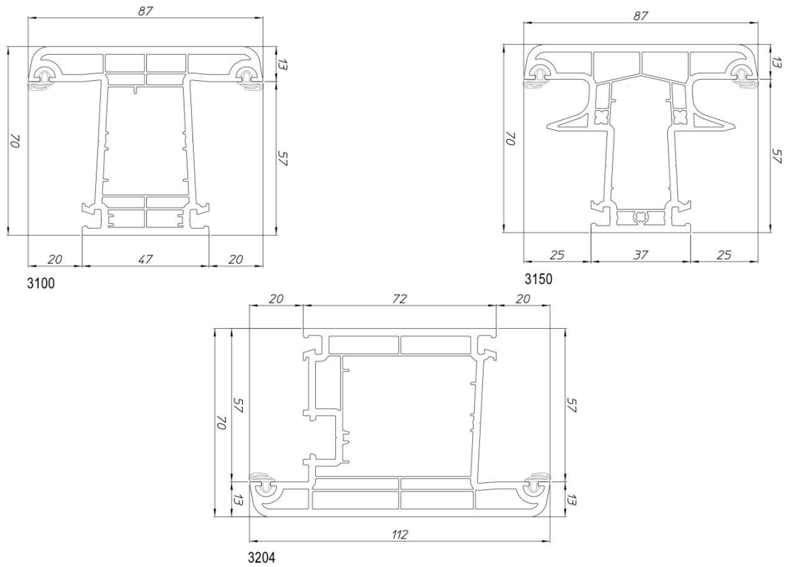
Figuur 4 – Weerstandsp profielen – makelaar
