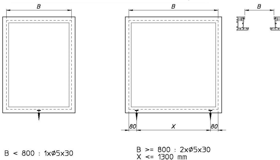
Figuur 10: ontluchting (drukvereffening) en afwatering
