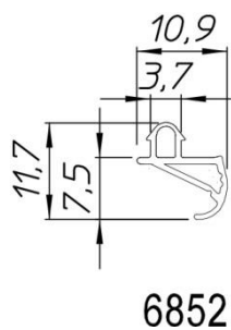
Figuur 6a – Aanslagdichtingen en glasdichting
