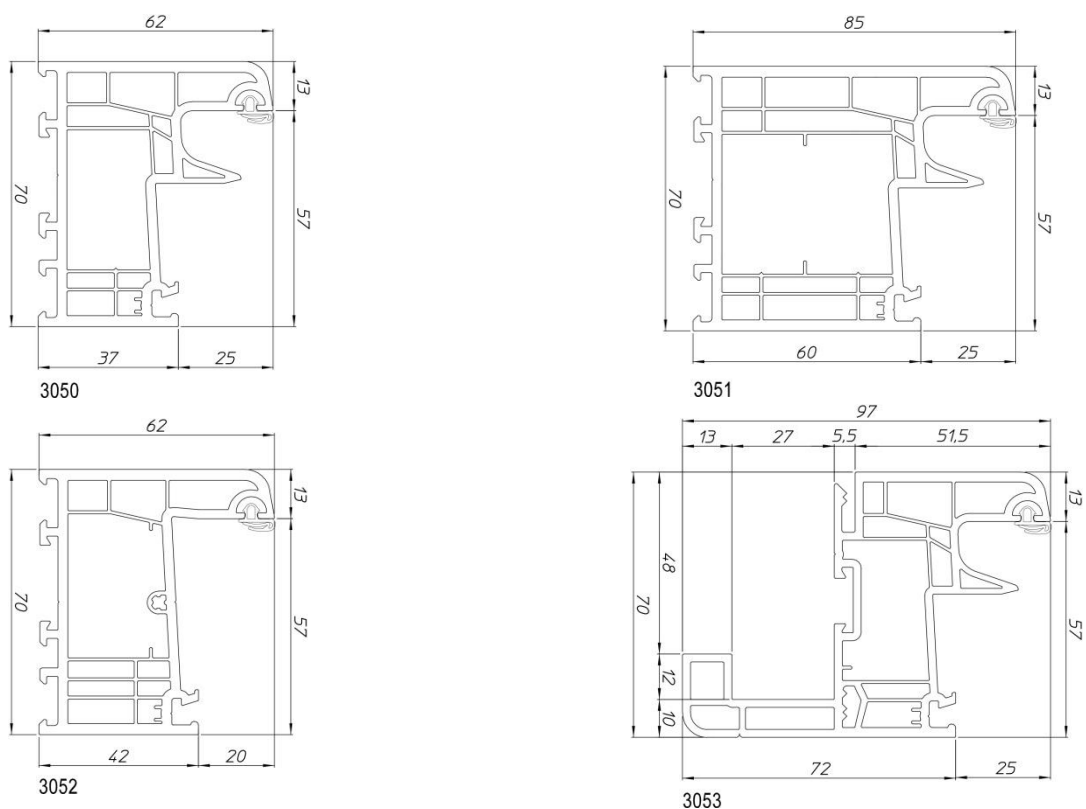
Figuur 2 – Weerstandsp profielen – vleugel
