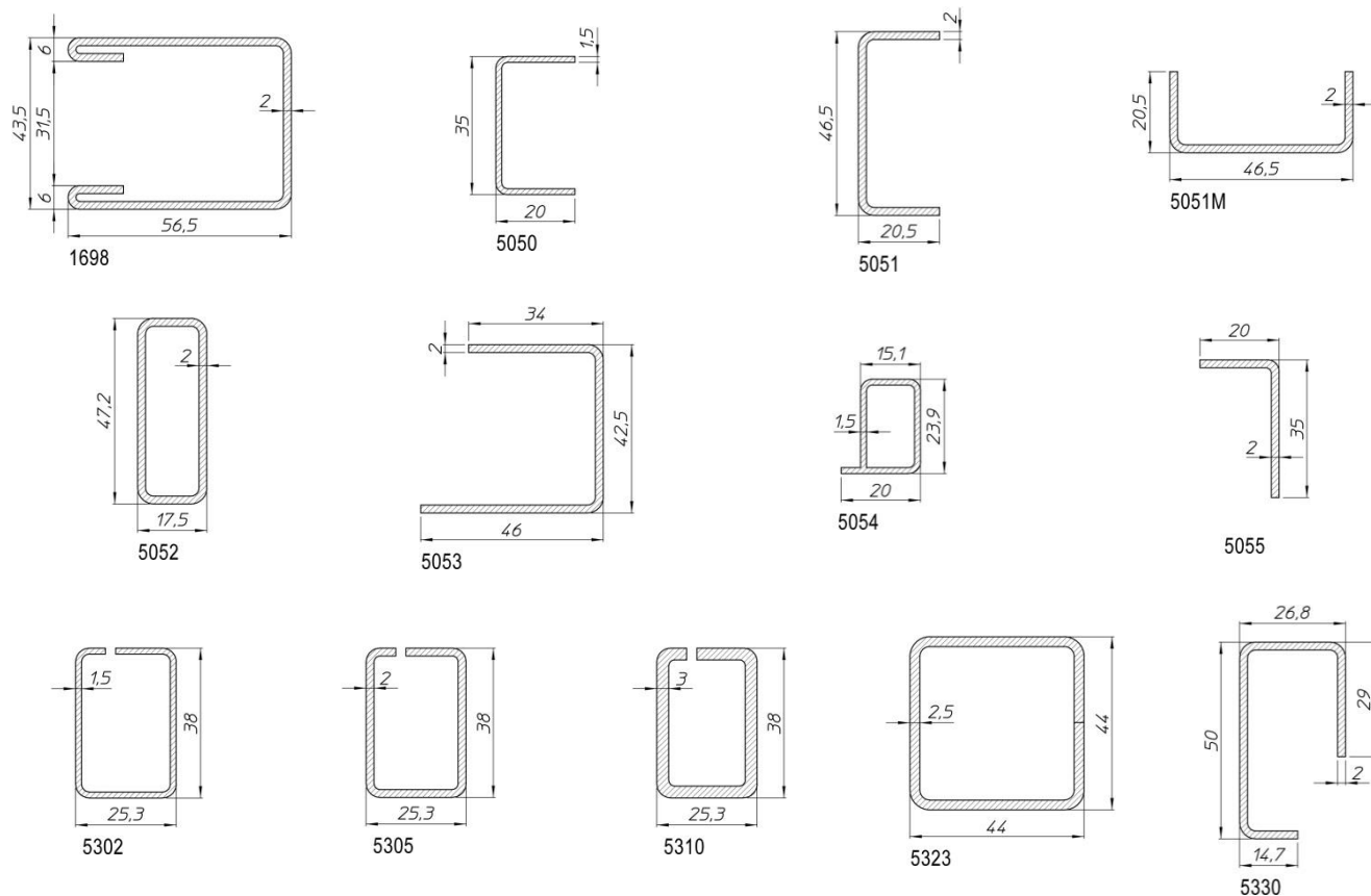
Figuur 5 – Versterkingsprofielen
