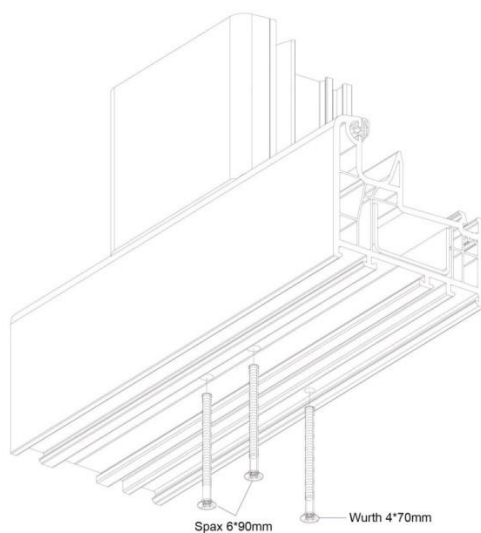
Figuur 7b – schroefverbinding
