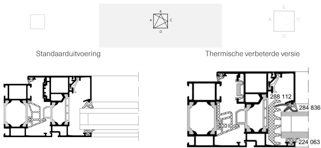
Figuur 3: Typesnede buitendraaiend venster
