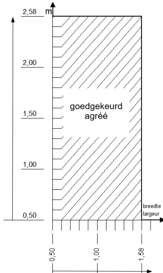
Beslagdiagramma
