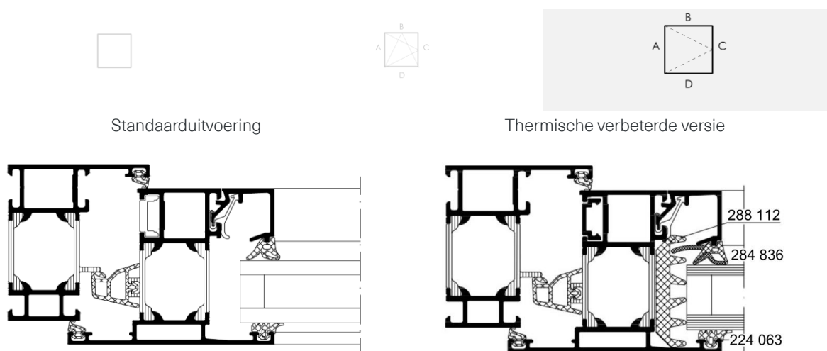
Figuur 3: Typesnede buitendraaiend venster
