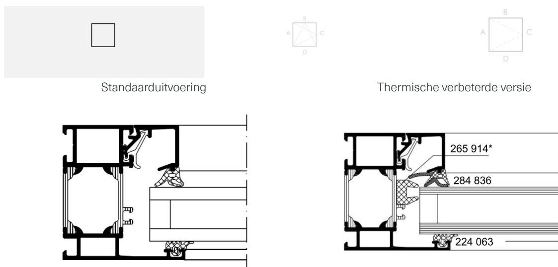
Figuur 2: Typesnede binnendraaiend venster draai-kipvenster
