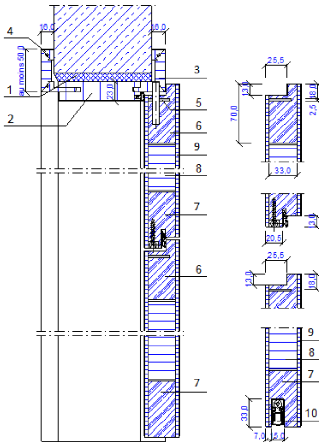
Figure 5 – Coupe verticale – avec imposte
