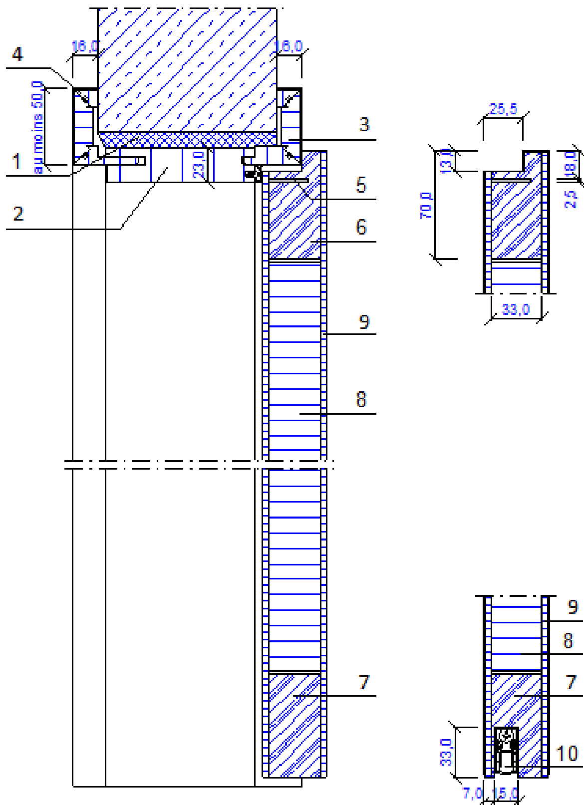
Figuur 1 – Verticale snede – zonder bovenpaneel - Type A
