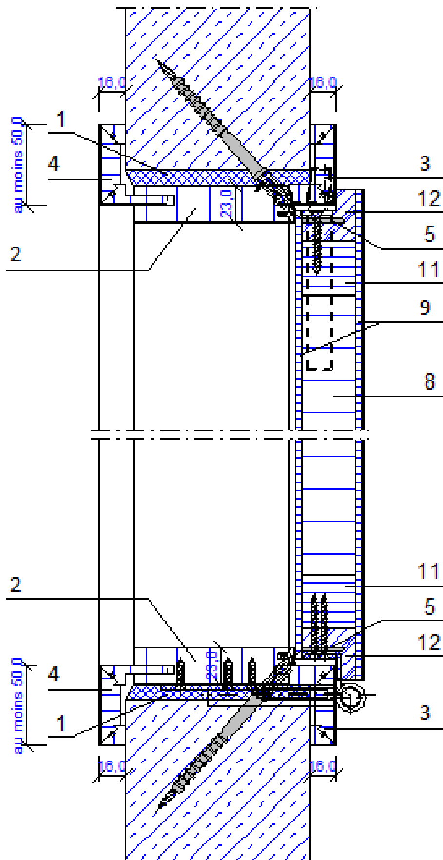
Figuur 2 - Horizontale snede - Type A
