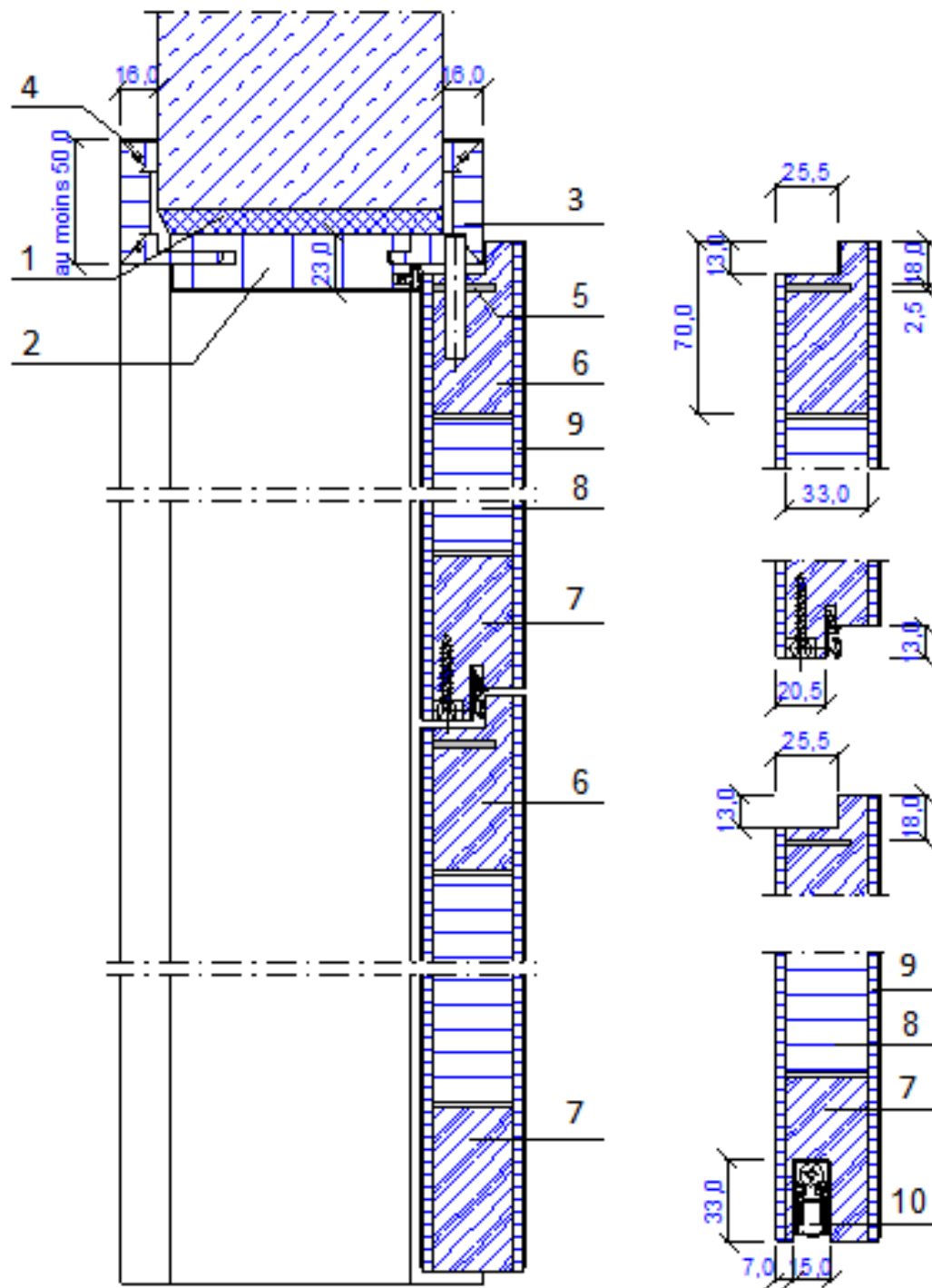
Figuur 5 – Verticale snede – met bovenpaneel
