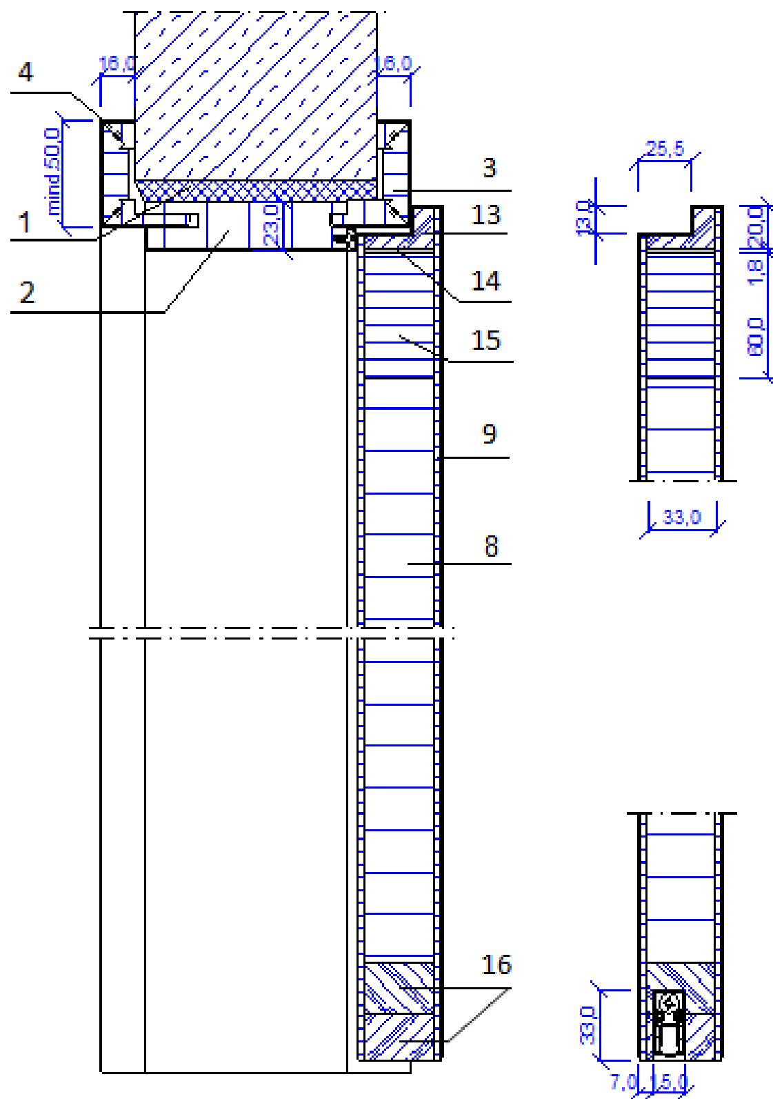
Figuur 3 – Verticale snede – zonder bovenpaneel - Type B
