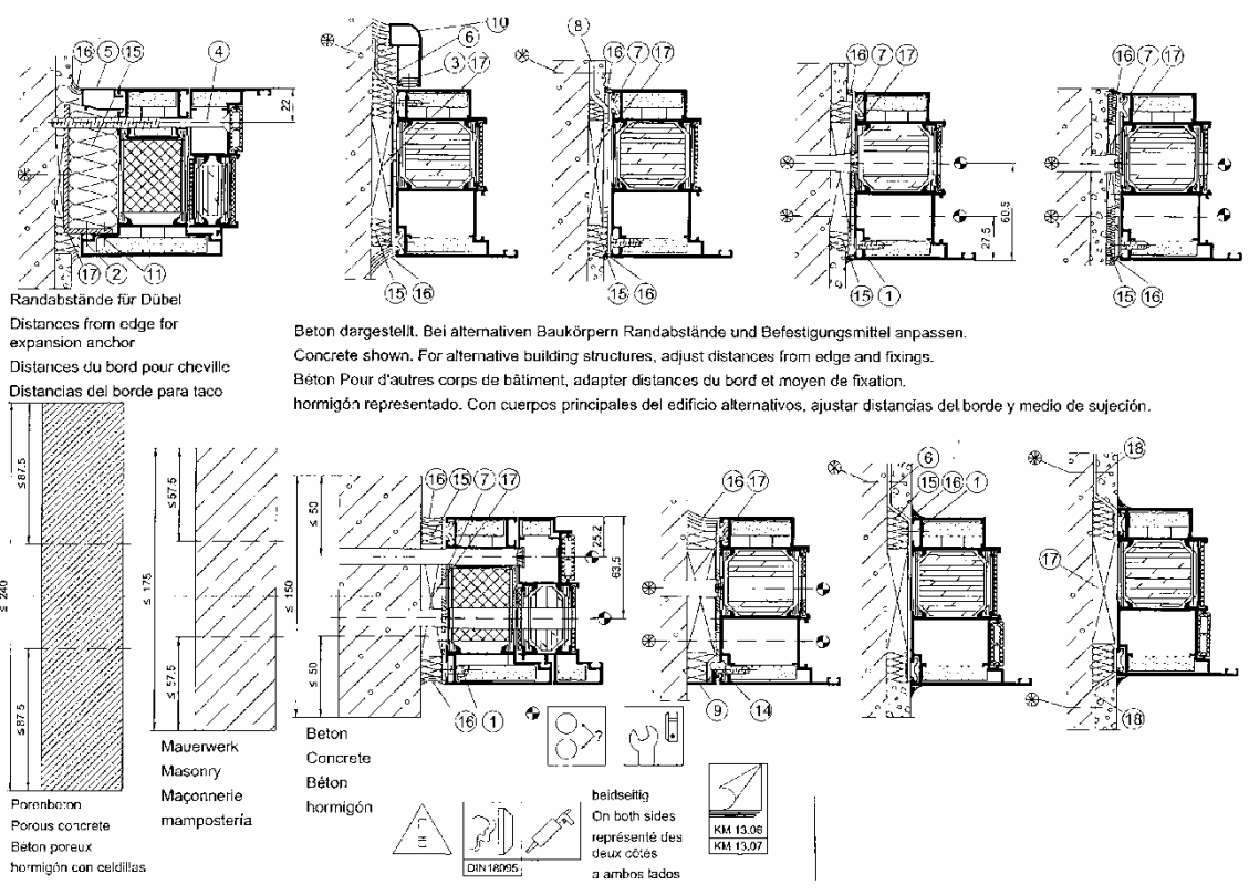
Figuur 8a: Wandaansluiting
