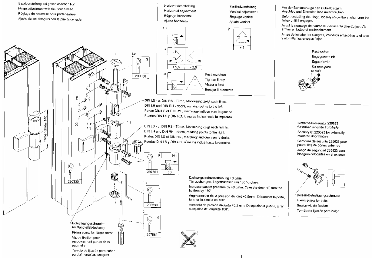
Figur 9d: Montage scharnieren
