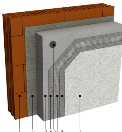
1. Support ; 2. Colle ; 3. Isolant ; 4. Enduit de base ; 5. (éventuelle) fixation mécanique ; 6. Tissu d'armature ; 7. Enduit de finition.
