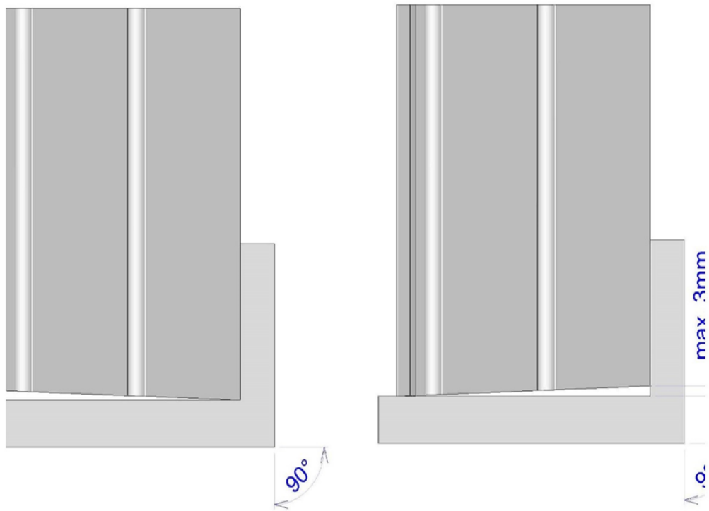
figuur 3: Controle van de haaksheid van de zaagsneden.
