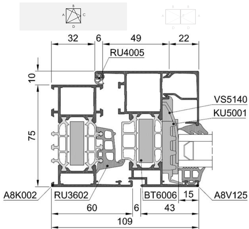
Figure 4 : Coupe-type de fenêtre oscillo-battante
