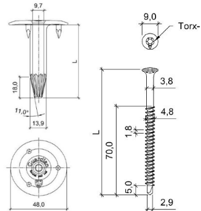
Fig. 3 – Schroef GUARDIAN BS 4,8 + tule GUARDIAN RB 48
