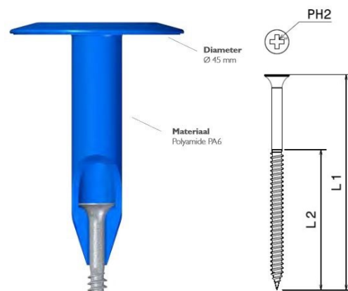
Fig. 4 – Schroef EUROFAST EDS-S 4,8 + EUROFAST TRP 45
