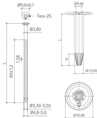
Fig. 1 – Schroef GUARDIAN PS 4,8 + bevestigingsplaatje R(P)45
