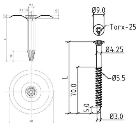
Fig. 6 – Schroef GUARDIAN BS 5,5 + bevestigingsplaatje GUARDIAN GWSP-80-F2E
