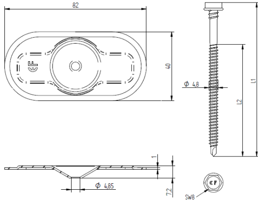
Fig. 5 – Schroef EUROFAST EDS-S 4,8 + EUROFAST TRP 45
