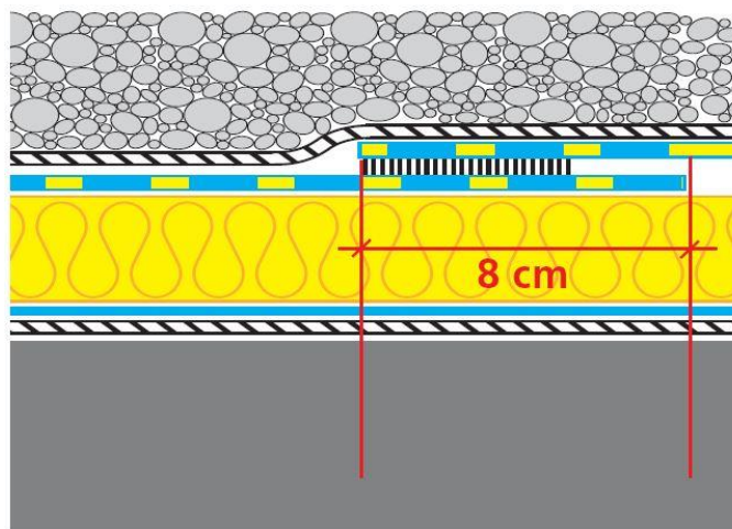
Fig. 9 – Langsnaad in losliggend systeem met ballast
