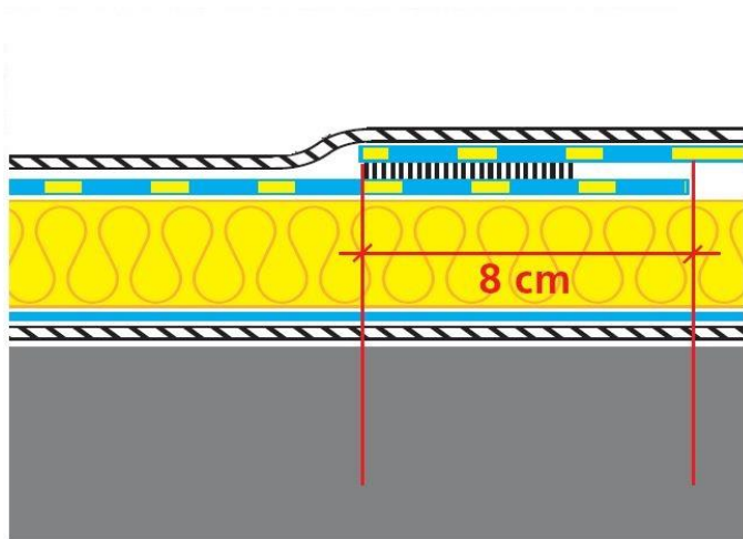
Fig. 10 – Langsnaad in verlijmd systeem en mechanisch bevestigd systeem met GUARDIANWELD/RHINO BOND
