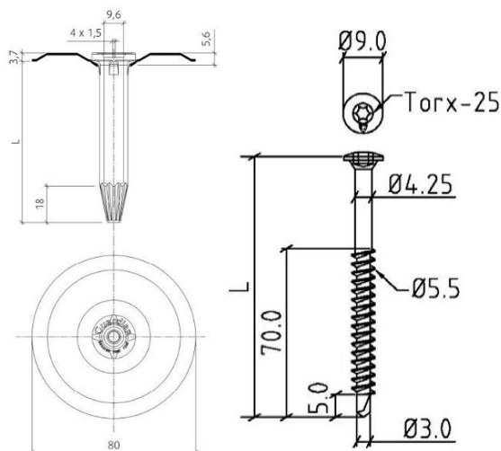
Fig. 6 – Schroef GUARDIAN BS 5,5 + bevestigingsplaatje GUARDIAN GWSPP-80-F2E
