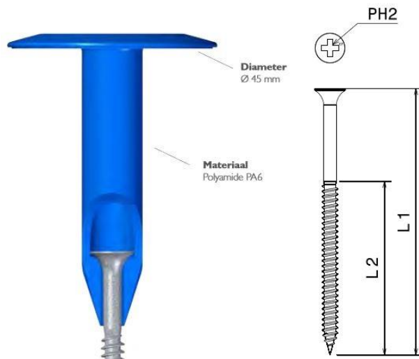
Fig. 4 – Schroef EUROFAST EDS-S 4,8 + EUROFAST TRP 45
