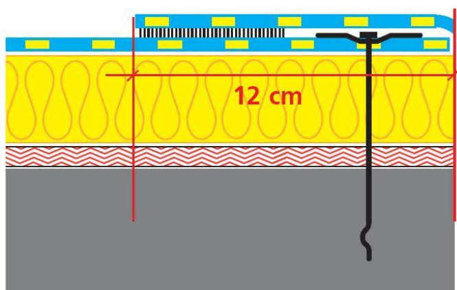
Fig. 11 – Langsnaad in een systeem met mechanisch bevestiging in de overlap
