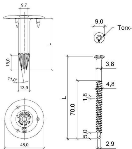
Fig. 3 – Schroef GUARDIAN BS 4,8 + tule GUARDIAN RB 48
