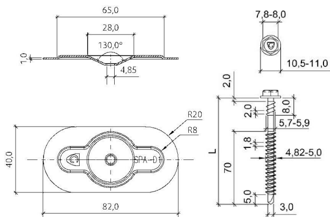
Fig. 4 – Schroef GUARDIAN DBT(A) + bevestigingsplaatje GUARDIAN SPA 82x40
