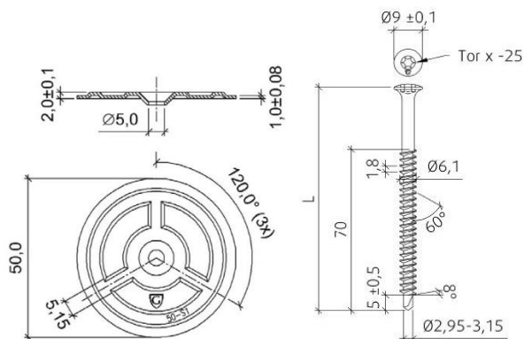
Fig. 3 – Schroef GUARDIAN PS 4,8 + bevestigingsplaatje GUARDIAN SP 50 S
