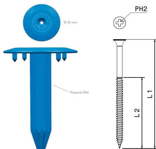
Fig. 2 – Schroef EUROFAST EDS-S 4,8 + EUROFAST BTRP 45
