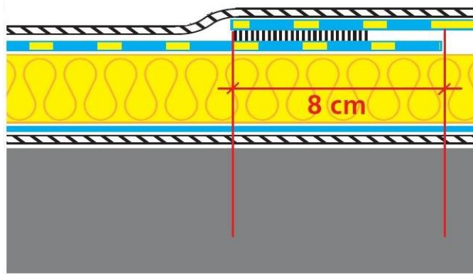
Fig. 10 – Langsnaad in verlijmd systeem en mechanisch bevestigd systeem met GUARDIANWELD
