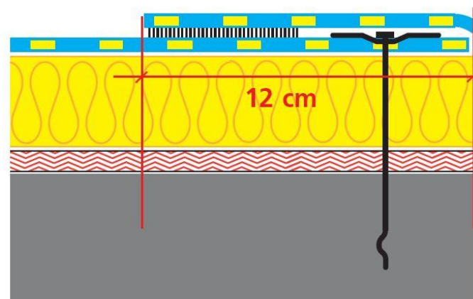
Fig. 11 – Langsnaad in een mechanisch bevestigd systeem
