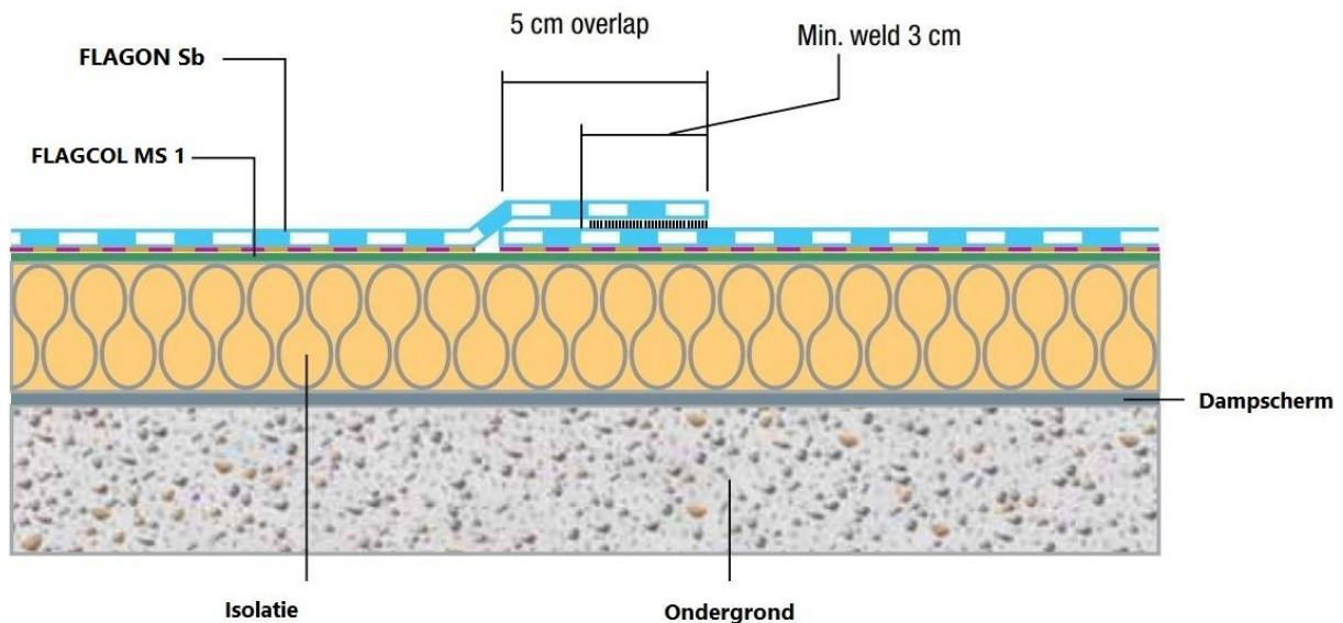
Fig. 12 – Langsnaad in verlijmd systeem
