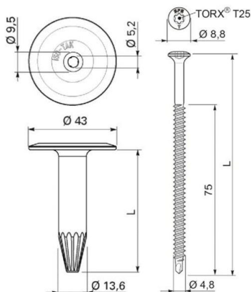
Fig. 6 – Schroef SFS BS 4,8 + Tule (ISO-TAK) RP 45
