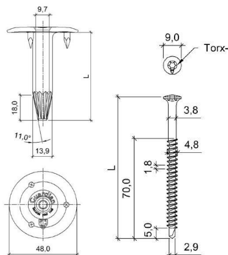
Fig. 5 – Schroef GUARDIAN BS 4,8 + tule GUARDIAN RB 48
