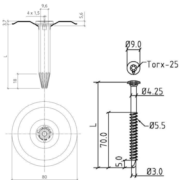
Fig. 7 – Schroef GUARDIAN BS 5,5 + bevestigingsplaatje GUARDIAN GWSPP-80-F2E
