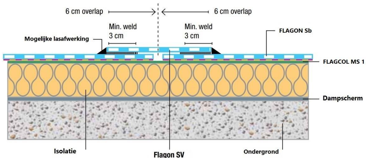
Fig. 13 – Dwarsnaad in verlijmd systeem
