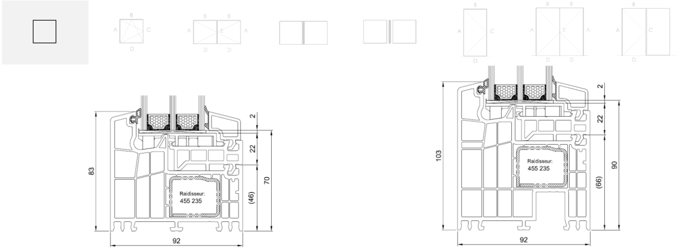
Figure 7a: Coupe-type de fenêtre fixe
