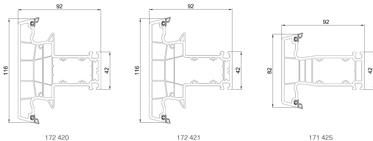
Figuur 2c: Tussenstijlen en dwarsregels
