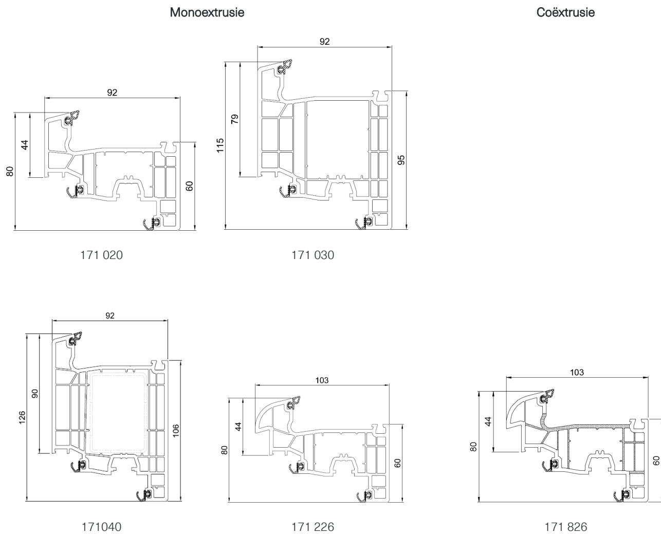
Figuur 2b: Vleugelprofielen
