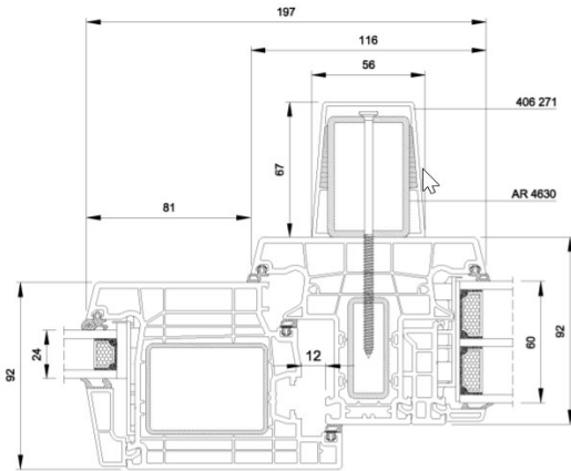
Doorsnede F/F
