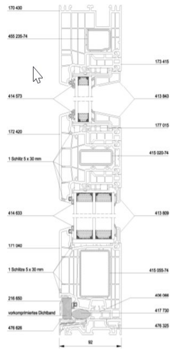
Doorsnede C/C
