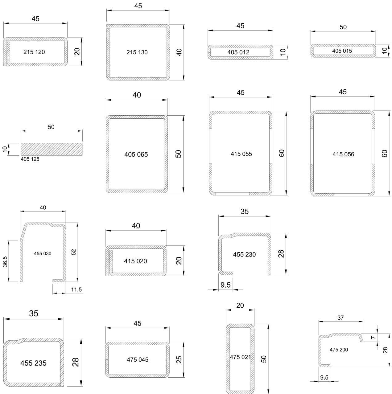
figuur 3: Versterkingsprofielen
