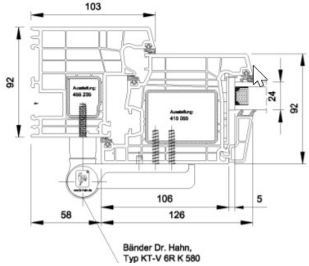
Doorsnede C/C
