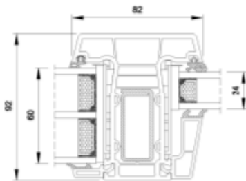
Doorsnede F/F
