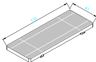
Figuur 6.a: Glassteunblokjes
