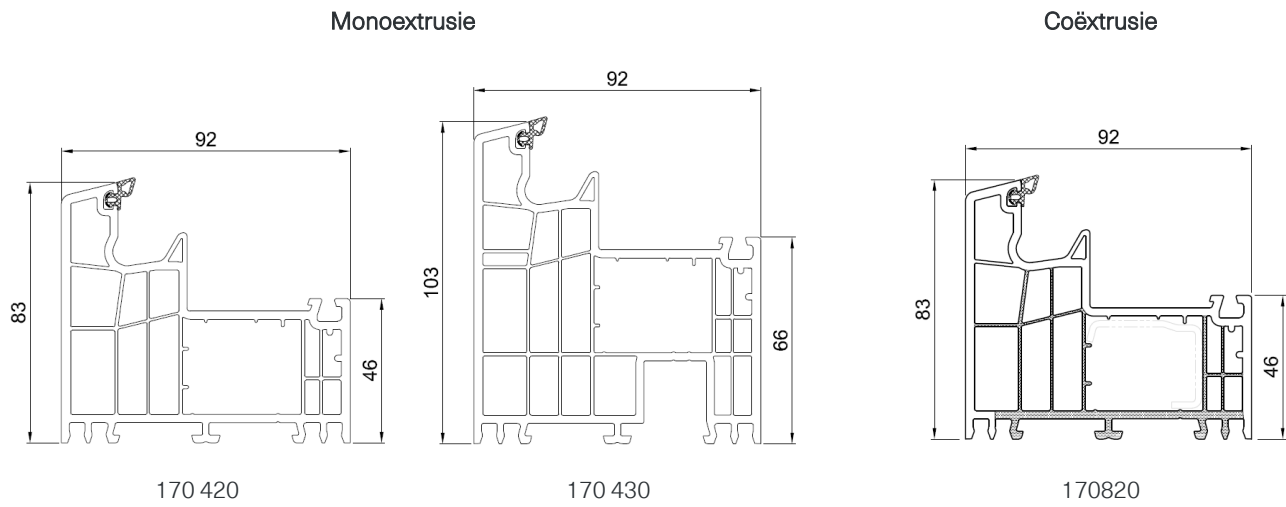
Figuur 2a: Kaderprofielen
