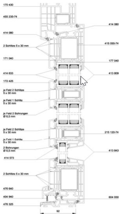
Doorsnede B/B
