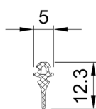
dichting 604930
