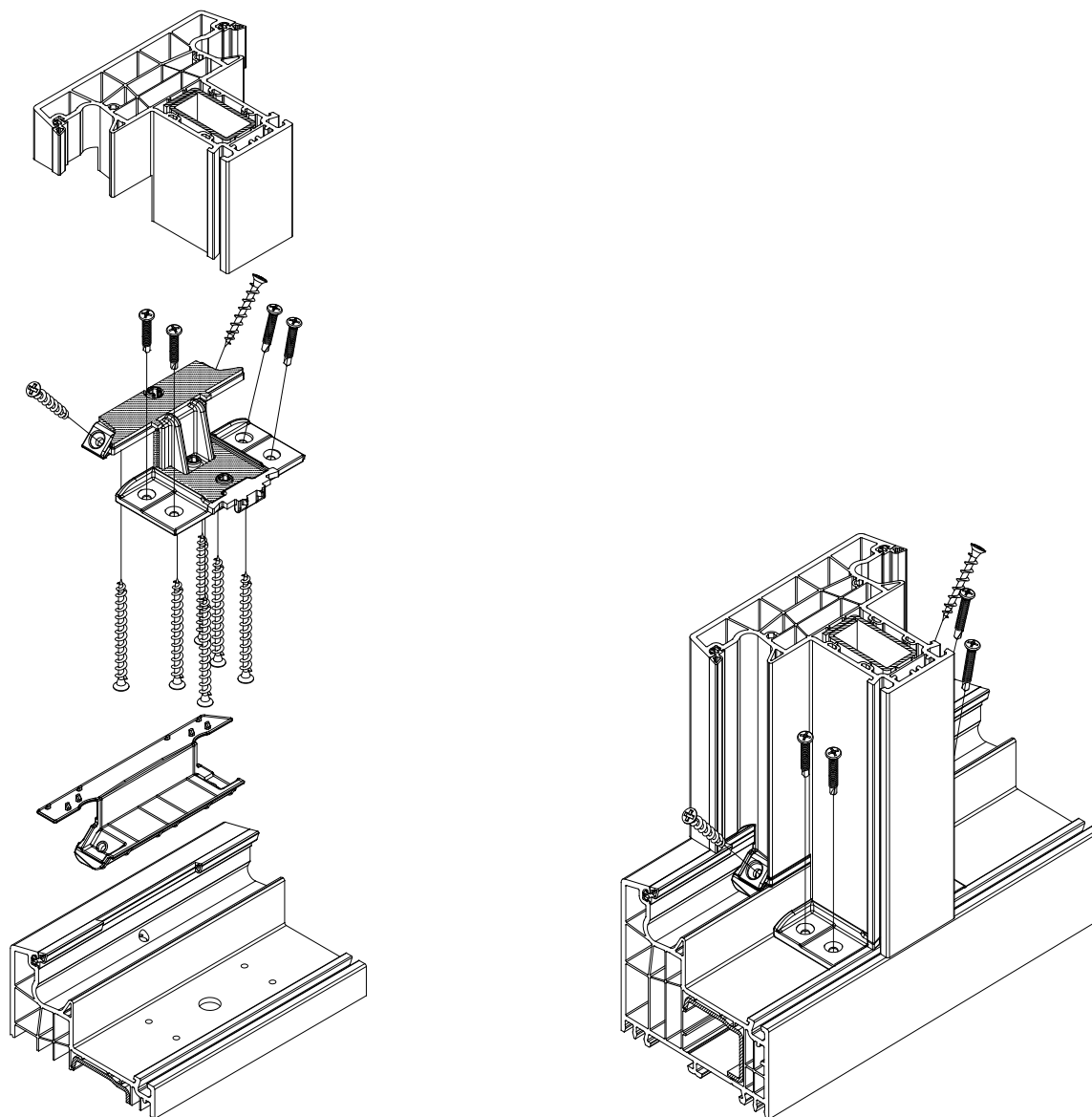
Figuur 2d: Mechanische T-verbinding
