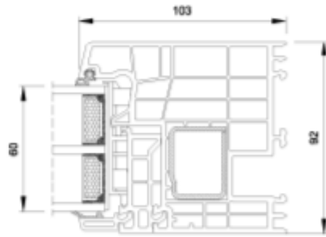
Doorsnede E/E
