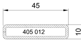
figuur 3: Versterkingsprofielen
