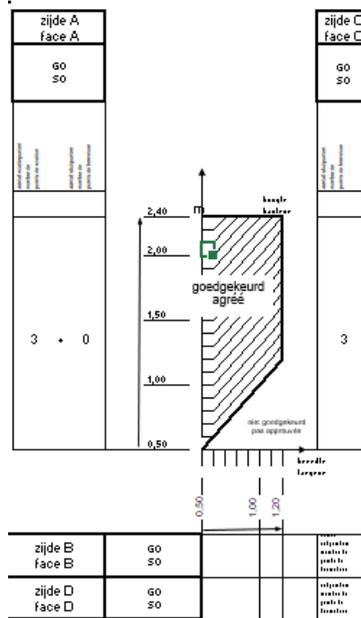
Beslagdiagram
