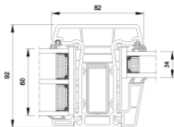
Doorsnede F/F
