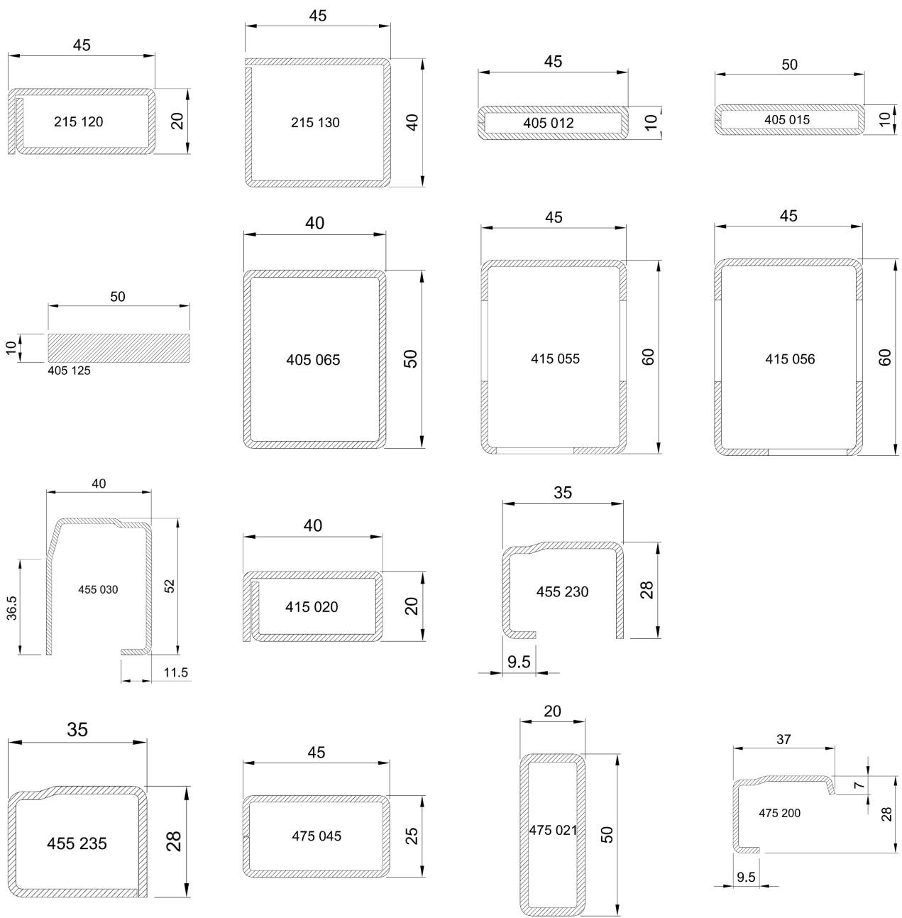
figuur 3: Versterkingsprofielen
