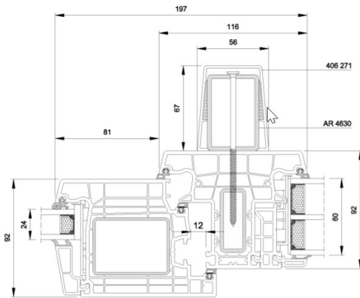
Doorsnede F/F
