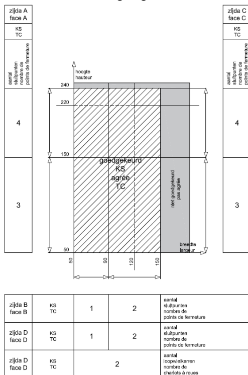
Beslagdiagram
