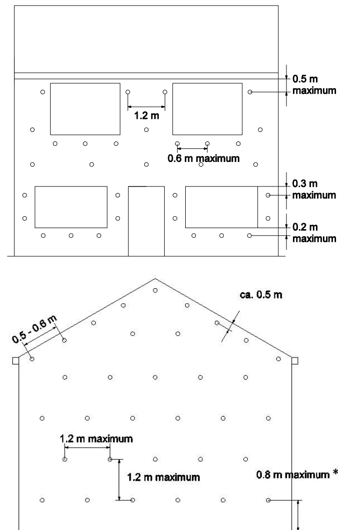
Figuur 1: Schematische weergave van het vulpatroon
