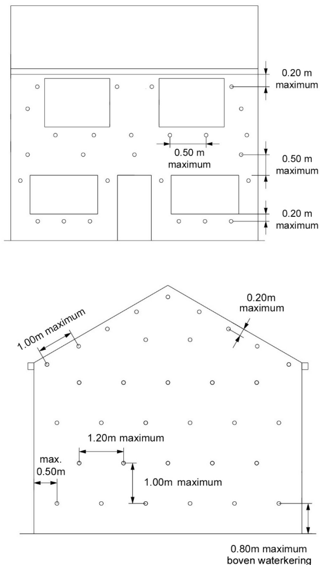
Fig. 1 Schematische weergave van het vulpatroon
