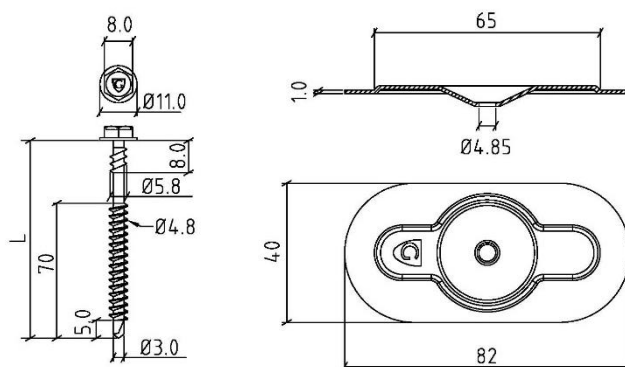
Fig. 4 – Schroef GUARDIAN DBT(A) 4,8 + bevestigingsplaatje GUARDIAN SPA 8240
