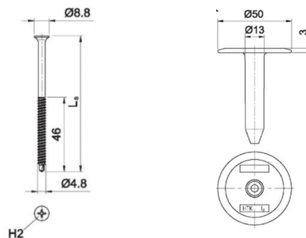
Fig. 6 – Schroef EJOT DABO® TKR 4,8 + telescopische tule EJOT HTK-2G 50
