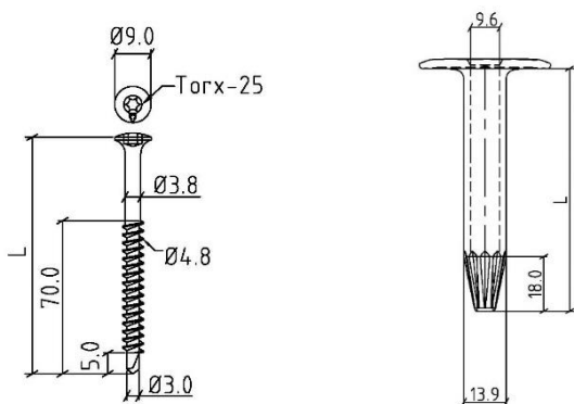
Fig. 2 – Schroef GUARDIAN BS 4,8 + telescopische tule GUARDIAN R 45
