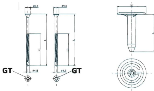
Fig. 8 – Schroef ETANCO GTS-B 4,8 + telescopische tule ETANCO G2 50
