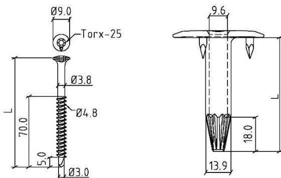
Fig. 3 – Schroef GUARDIAN BS 4,8 + telescopische tule GUARDIAN RB 48
