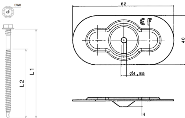
Fig. 5 – Schroef EUROFAST EDS-BZT + bevestigingsplaatje EUROFAST DVP-EFZK-8240D
