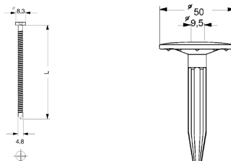
Fig. 7 – Schroef ZAHN ZDBK 4,8 + telescopische tule ZAHN ZKSH-R
