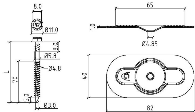
Fig. 4 – Schroef GUARDIAN DBT(A) 4,8 + bevestigingsplaatje GUARDIAN SPA 8240
