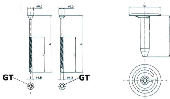
Fig. 8 – Schroef ETANCO GTS-B 4,8 + telescopische tule ETANCO G2 50
