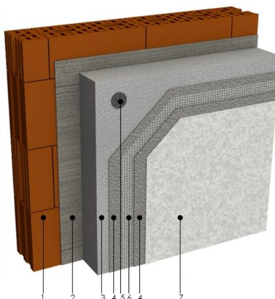
1. Support; 2. Adhésif; 3. Isolant; 4. Enduit de base; 5. (éventuelle) fixation mécanique; 6. Tissu d'armature; 7. Enduit de finition.
