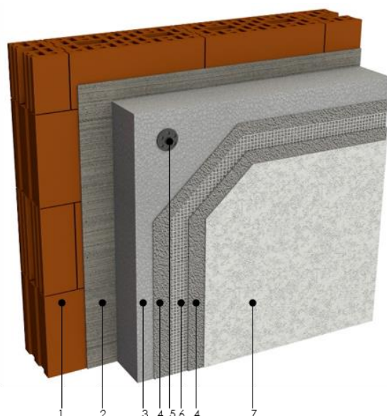
1. Support; 2. Adhésif; 3. Isolant; 4. Enduit de base; 5. (éventuelle) fixation mécanique; 6. Tissue d'armature; 7. Enduit de finition.
