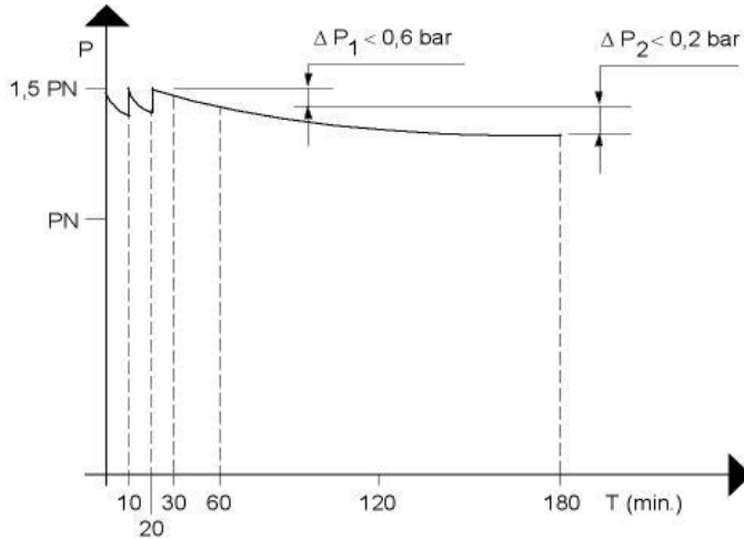
Figure 1 — Contrôle d'étanchéité
