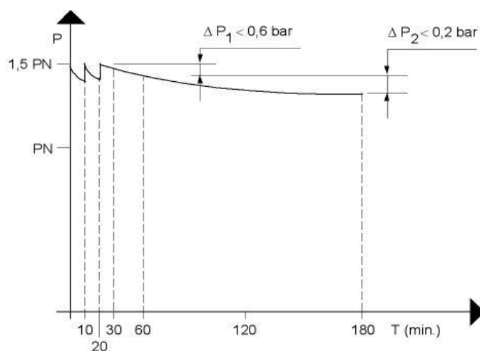
Figure 1 — Contrôle d'étanchéité
