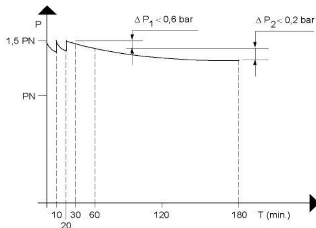
Fig. 3: Dichtheidscontrole
