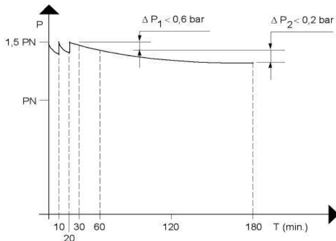
Figuur 1 — Dichtheidscontrole
