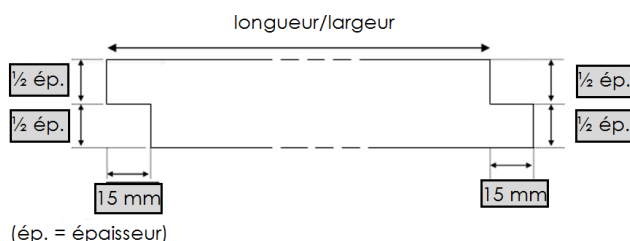
Fig. 1 – feuillure
