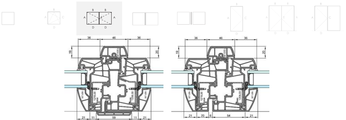
Figuur 7c: Typesnede dubbel opendraaiend venster met makelaar
