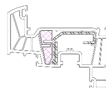
Profiel 1208 met versterking isolatiestrip 1208.62
