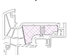
Profiel 1218 zonder versterking isolatiestrip 1208.61
