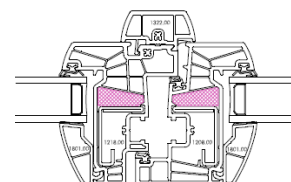
Si pas de renfort dans l'ouvrant
