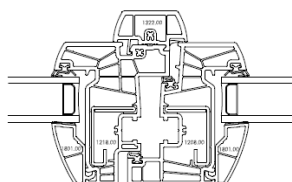
Variantes ensemble avec maclair ELITH PVC ISO
