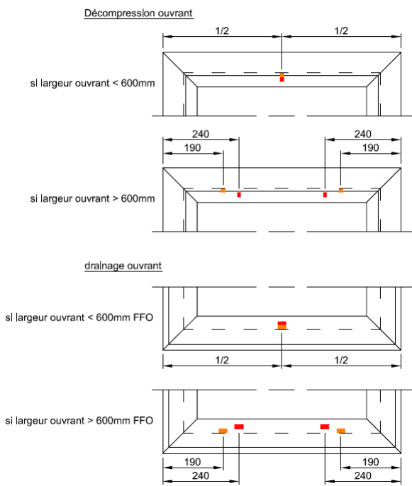
Figuur 8 (vervolg): Ontwatering en drukvereffening
