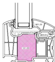
Varianten voor opendraaiend venster ELITH PVC ISO
