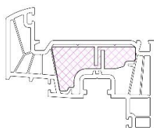
Profiel 1208 zonder versterking isolatiestrip 1208.61
