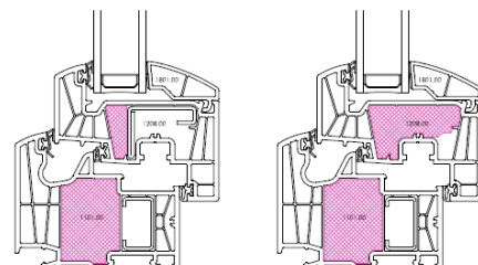
ELITH PVC A+++ Si renfort dans l'ouvrant Si pas de renfort dans l'ouvrant
