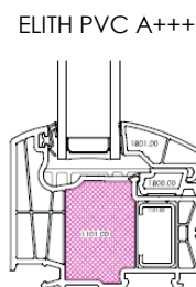
ELITH PVC A+++ Si renfort dans l'ouvrant Si pas de renfort dans l'ouvrant
