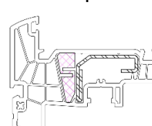
Profiel 1218 met versterking isolatiestrip 1208.62
