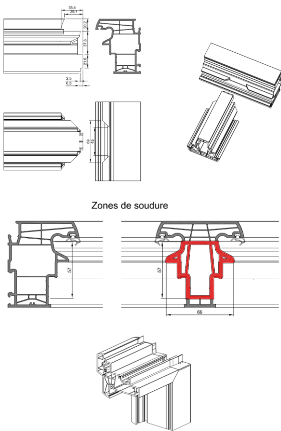
Figuur 2d.1: Verbinding van stijlen
