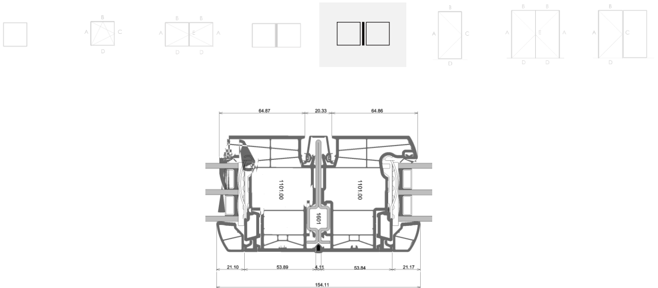
Figuur 7e : Typesnede schrijnwerkgeheel
