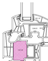
Variantes ensemble avec maclair ELITH PVC ISO
