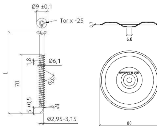
Fig. 3 – GUARDIAN BS 6,1 + plaquette GUARDIAN GWSPT-80-F2E
