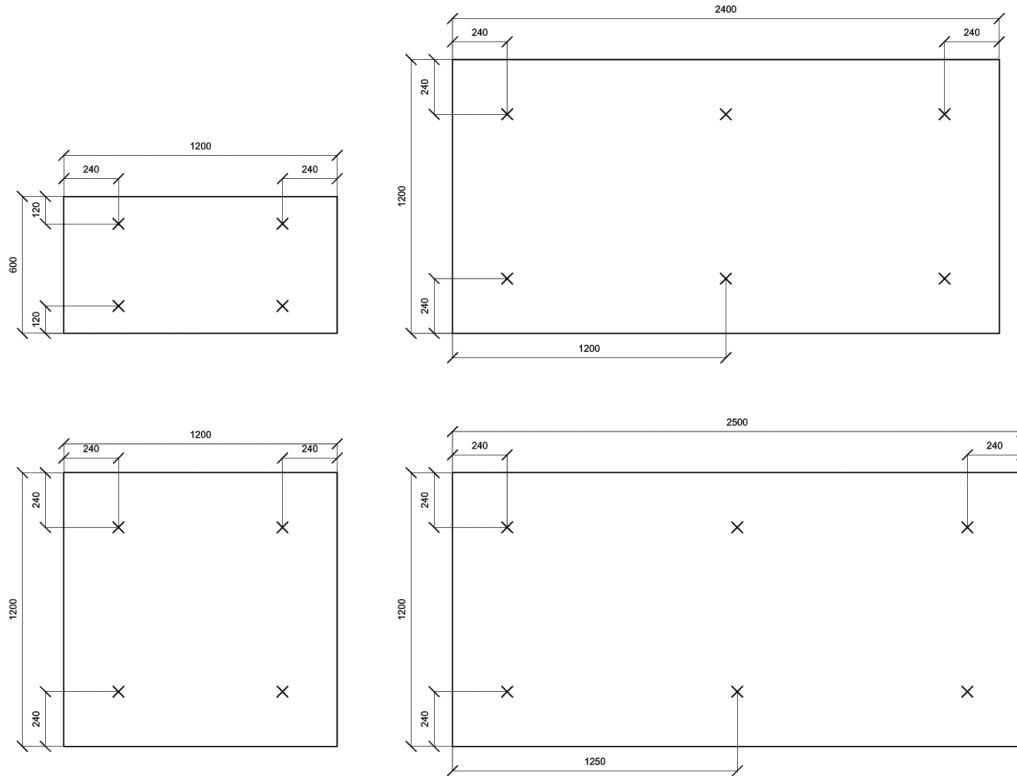
Fig. 1 – Plaatsingspatronen voor de mechanische bevestigingen
