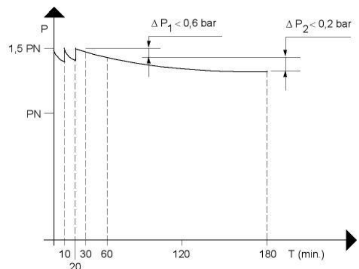
Figuur 5: procedure voor de dichtheidscontrole
