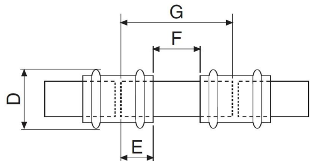
Figuur 2 : minimale afstanden tussen de fittingen
