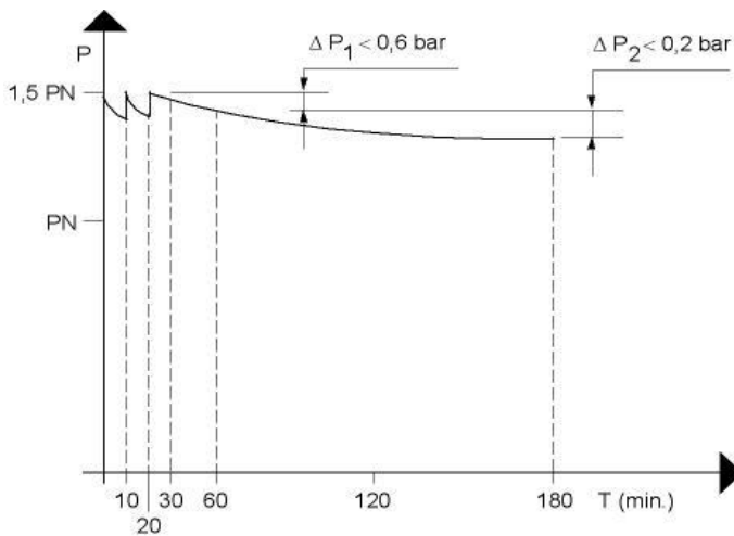
Figure 1 — Contrôle d'étanchéité
