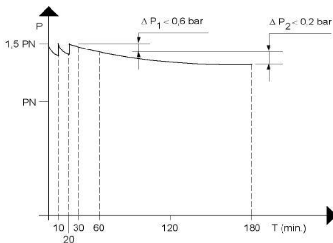
Figure 1 — Contrôle d'étanchéité
