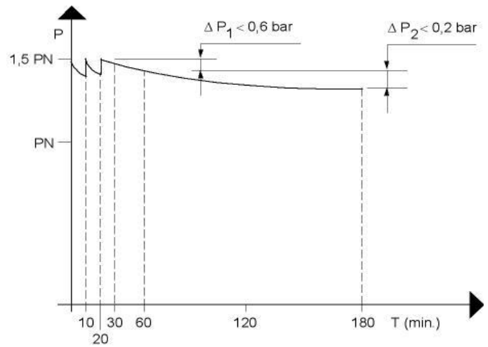
Figure 1 — Contrôle d'étanchéité
