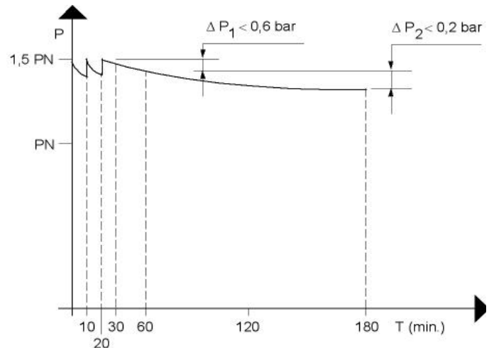
Figuur 1 — Dichtheidscontrole
