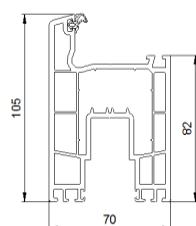
Figuur 2b: Vleugelprofiel
