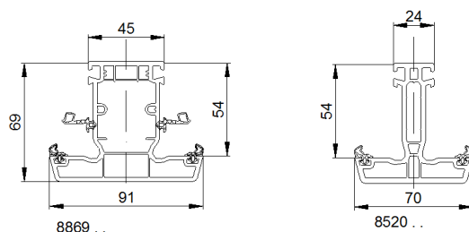
Figuur 3 – Versterkingsprofielen uit gegalvaniseerd staal
