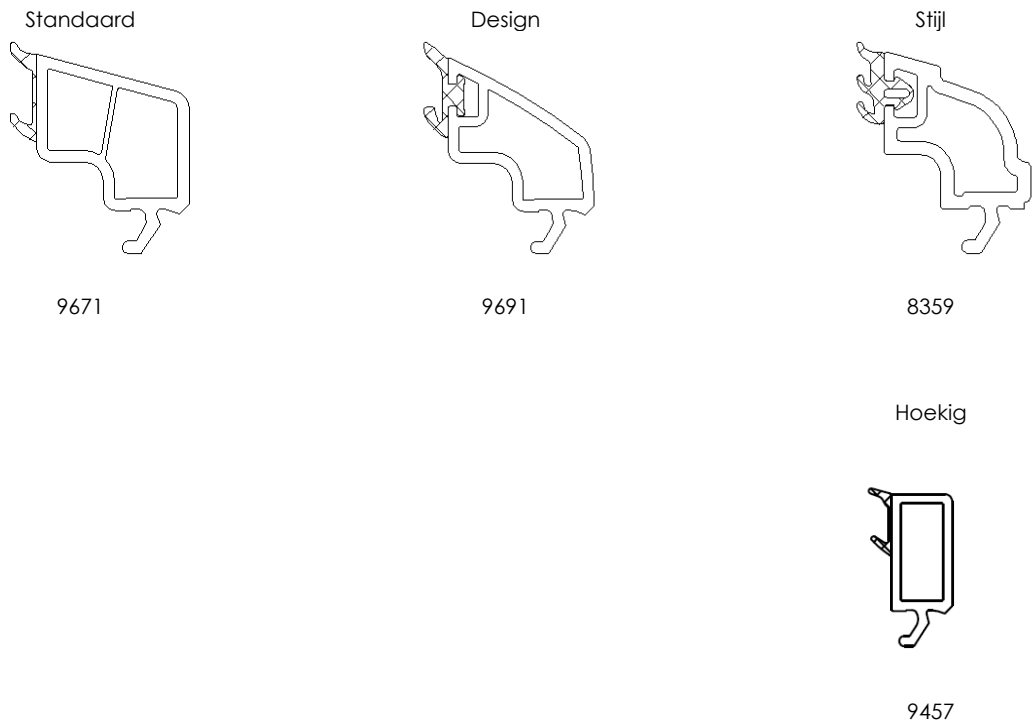
Figuur 5 : Uitvoeringsvarianten glaslatten
