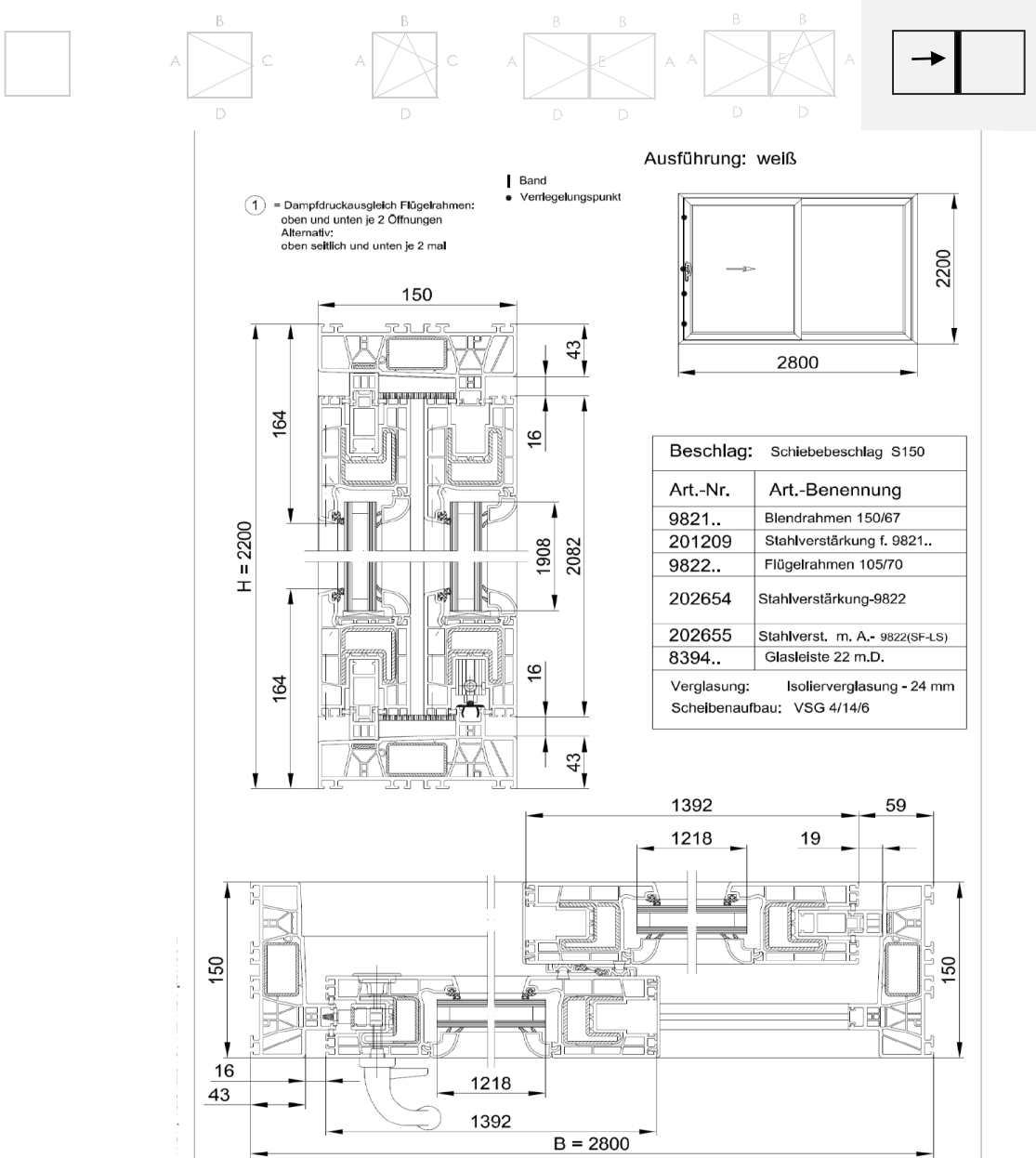
Figure 7: Coupes type de la fenêtre coulissante
