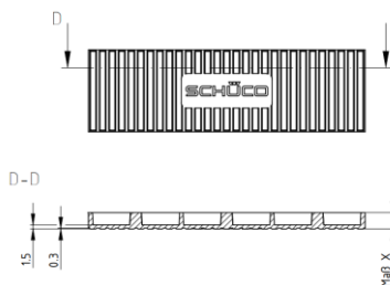
Figure 6d : Coiffe des ouvertures de drainage
