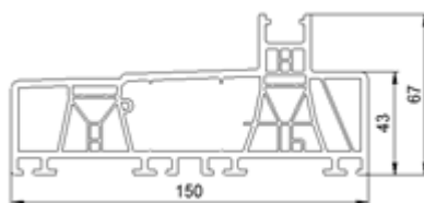
Figuur 2a: Kaderprofielen
