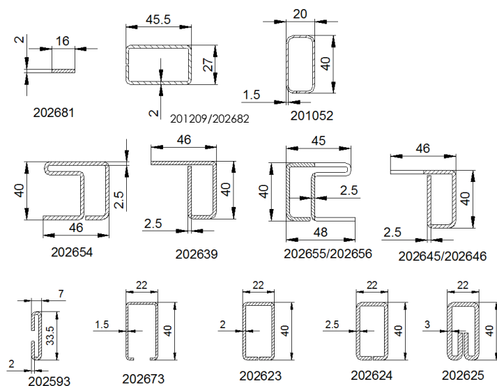
Figuur 3 – Versterkingsprofielen uit gegalvaniseerd staal
