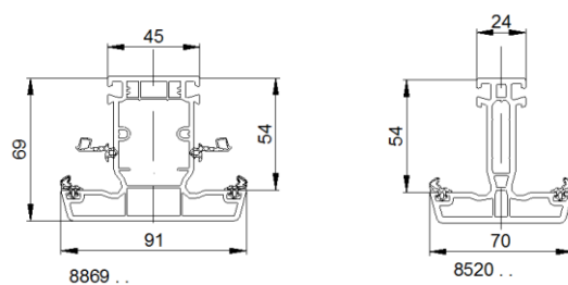
Figuur 3 – Versterkingsprofielen uit gegalvaniseerd staal
