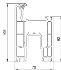
Figuur 2b: Vleugelprofiel
