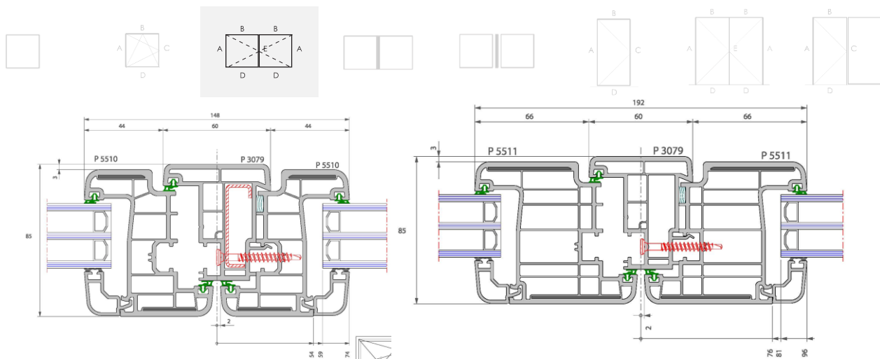
Figuur 2d: Typesnede van naar binnen opengaand draai-kipvenster met dubbele vleugel en eventueel staalversterkte makelaar op draivleugel
