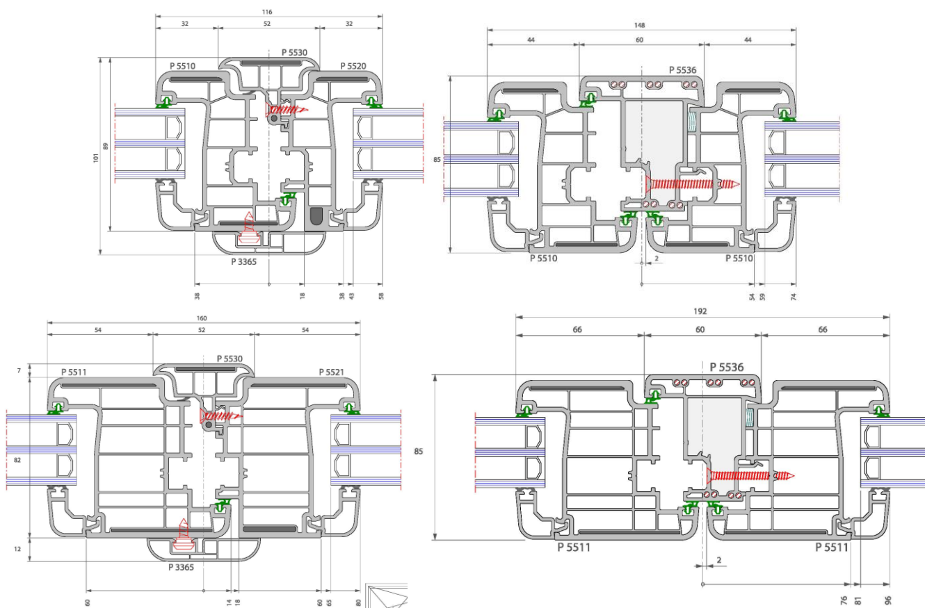
Figuur 2d: Typesnede van naar binnen opengaand draai-kipvenster met dubbele vleugel en eventueel staalversterkte makelaar op draivleugel
