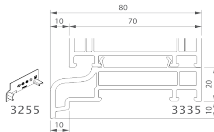
Figuur 7: Raamdorpel
