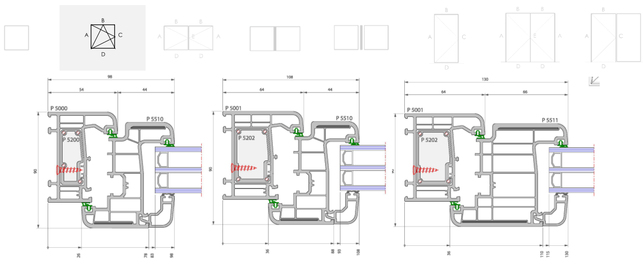
Figuur 2b: Typesnede draai-kip venster
