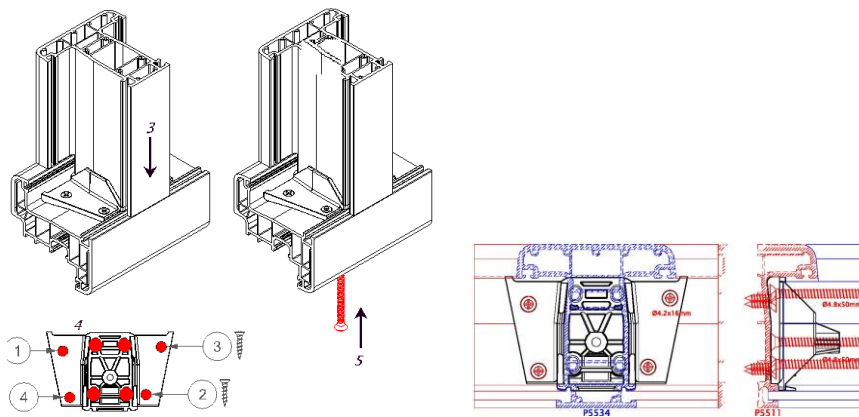
Figuur 5: Mechanische T-verbinding
