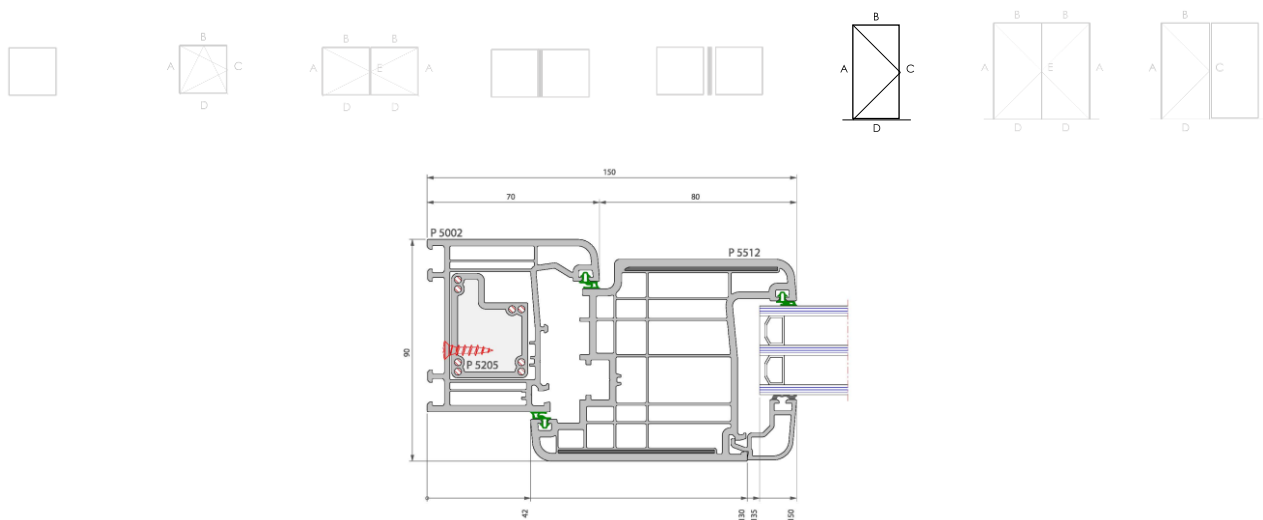
Figuur 2c: Typesnede deur
