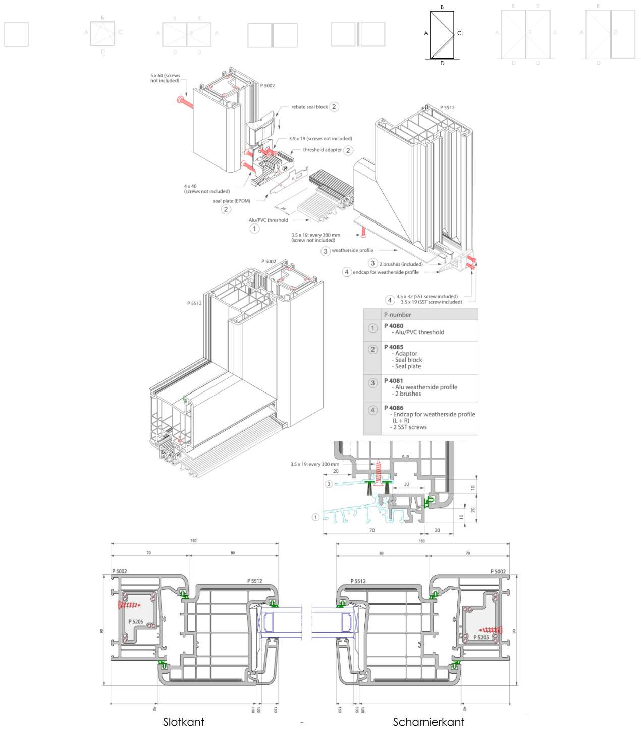
Figuur 3: Typesnede van naar binnen opengaande deur
