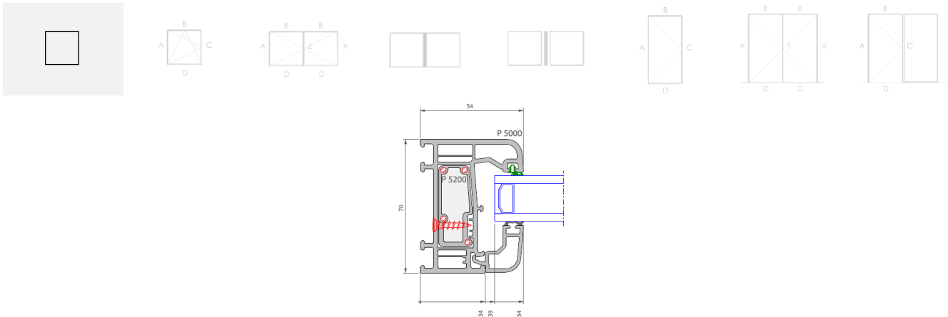
Figuur 2a: Typesnede vast venster (kader voor vast venster behoort tot ATG 2970)
