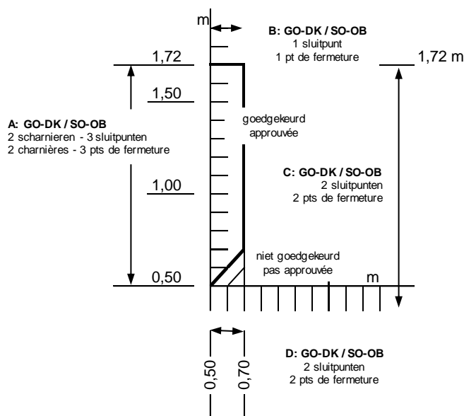
Beslagdiagram
