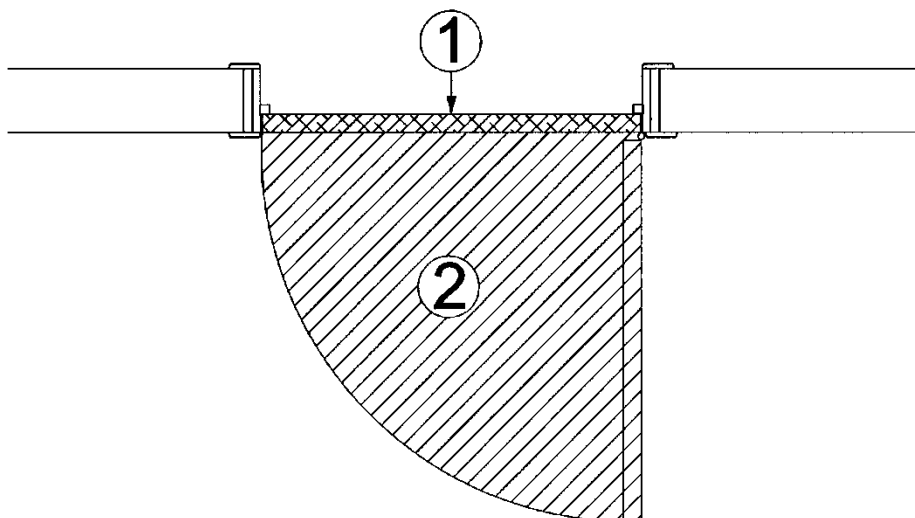
Fig. 15 positie silicone
