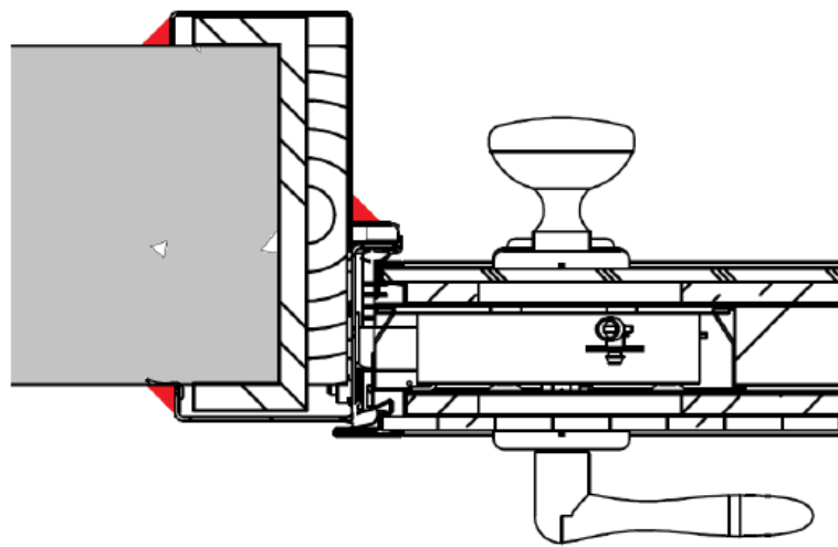
Fig. 15 positie silicone
