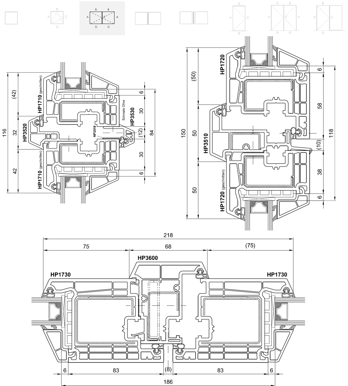
Figure 7c: Coupe-type de fenêtre à double ouvrant avec mauclair
