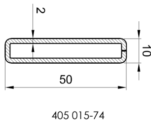
Figure 3: Profilés de renfort
