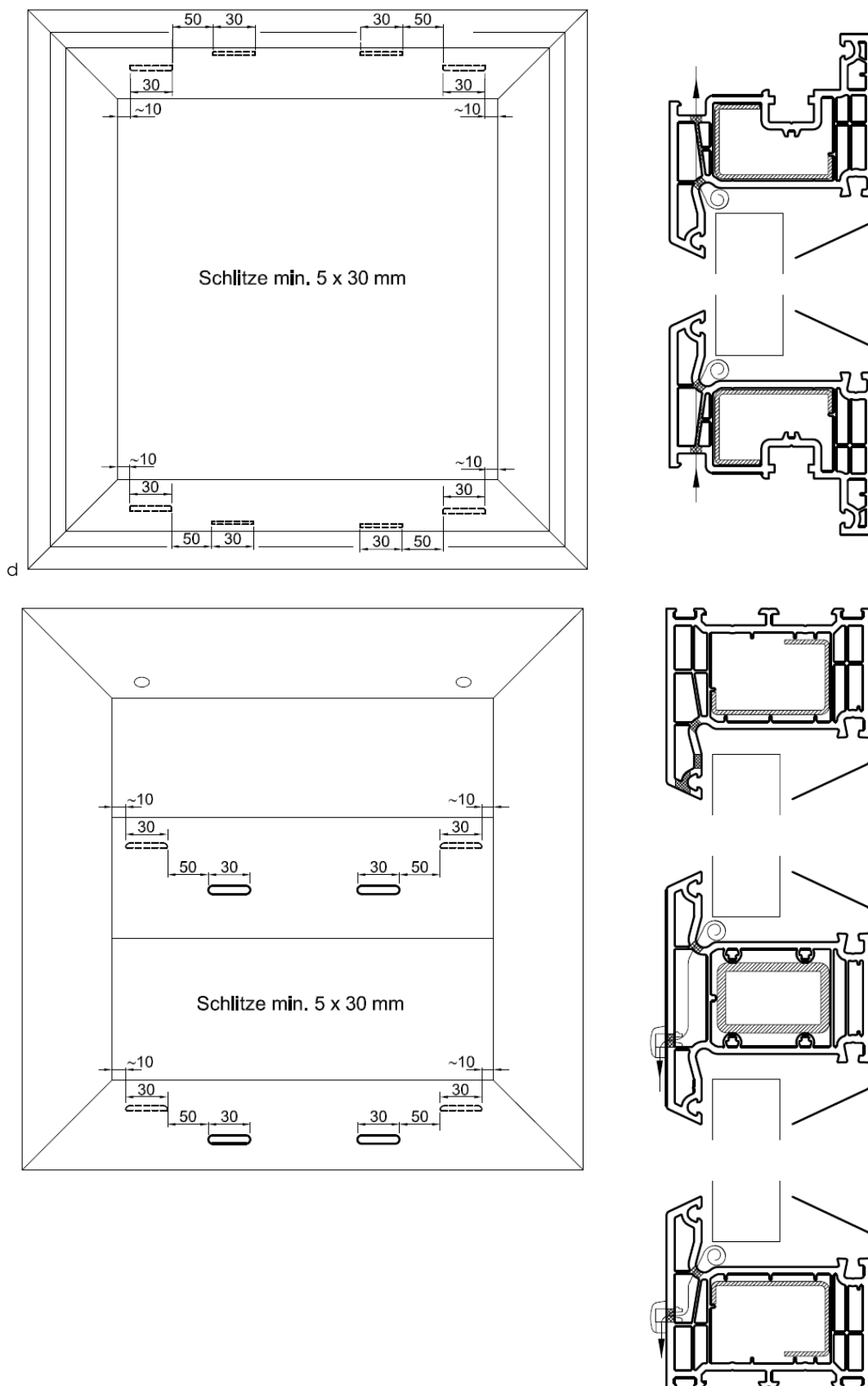
Figure 8b: Drainage et décompression
