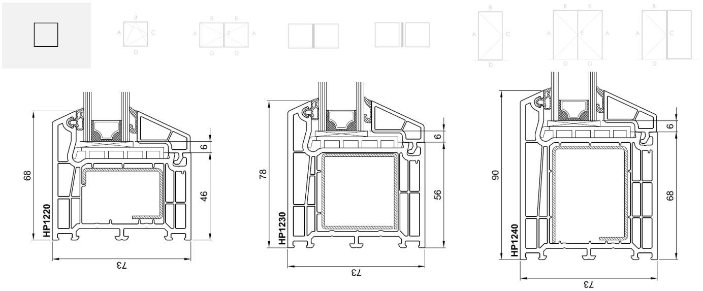
Figure 7b: Coupe-type de fenêtre oscillo-battante
