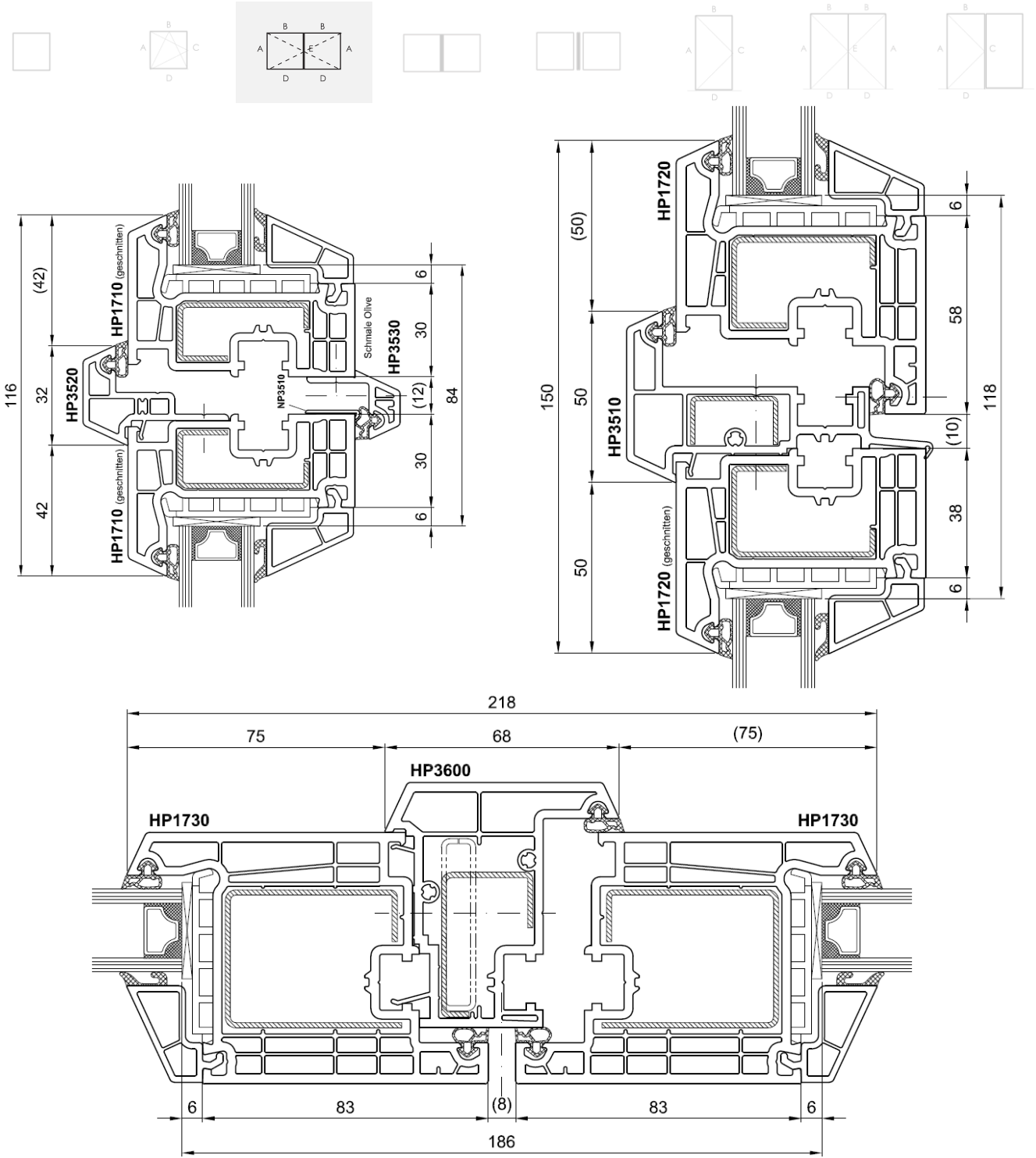
Figure 7c: Coupe-type de fenêtre à double ouvrant avec maucclair
