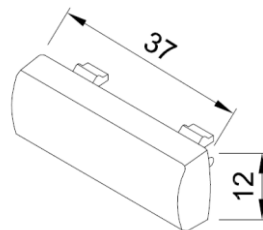
Figure 6d : coiffes pour ouvertures de drainage
