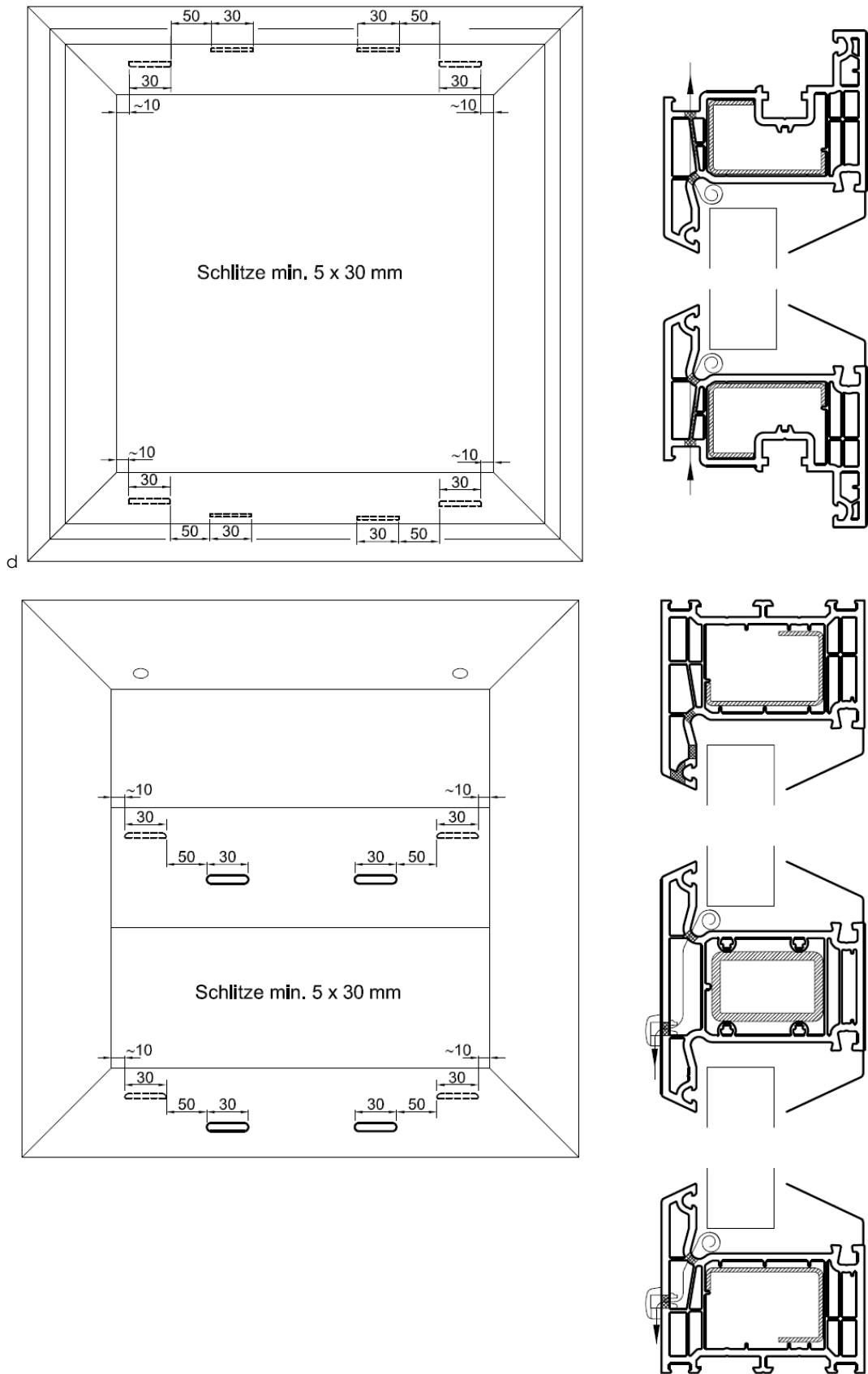
Figure 8b: Drainage et décompression
