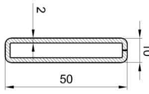
Figuur 3: Versterkingsprofielen
