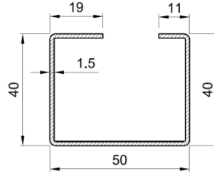
Figuur 3: Versterkingsprofielen
