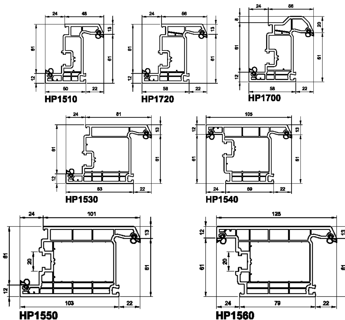
Figuur 2 – Weerstandprofielen – vleugel
