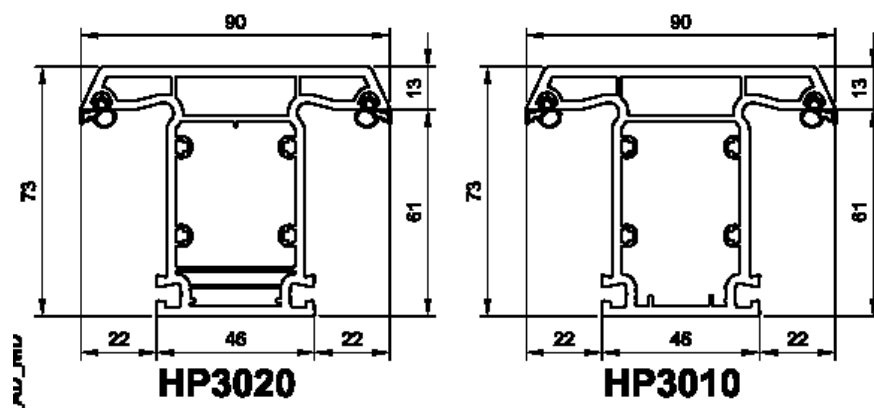
Figuur 4 – Versterkingsprofielen
