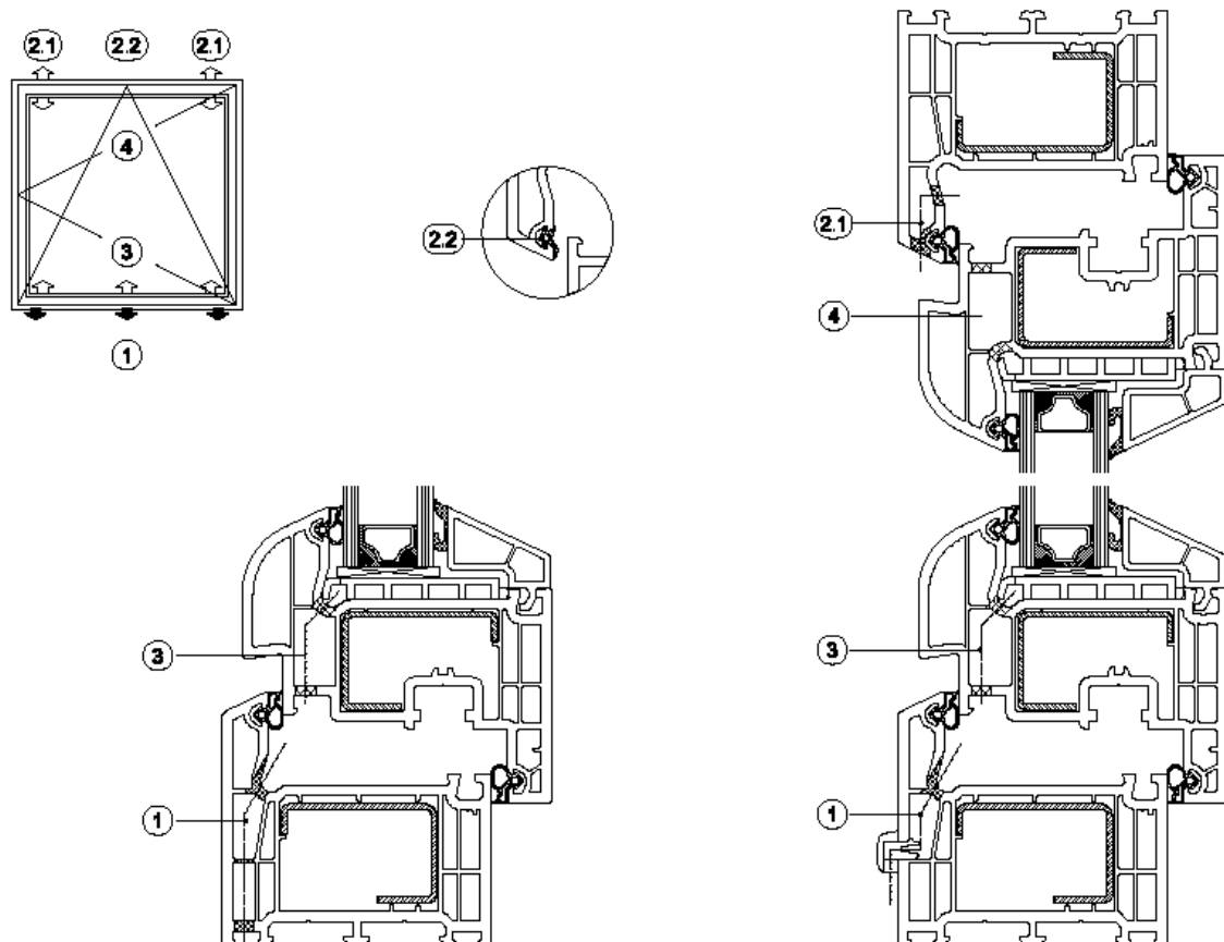
Figuur 11 – schema afwatering en ontluchting
