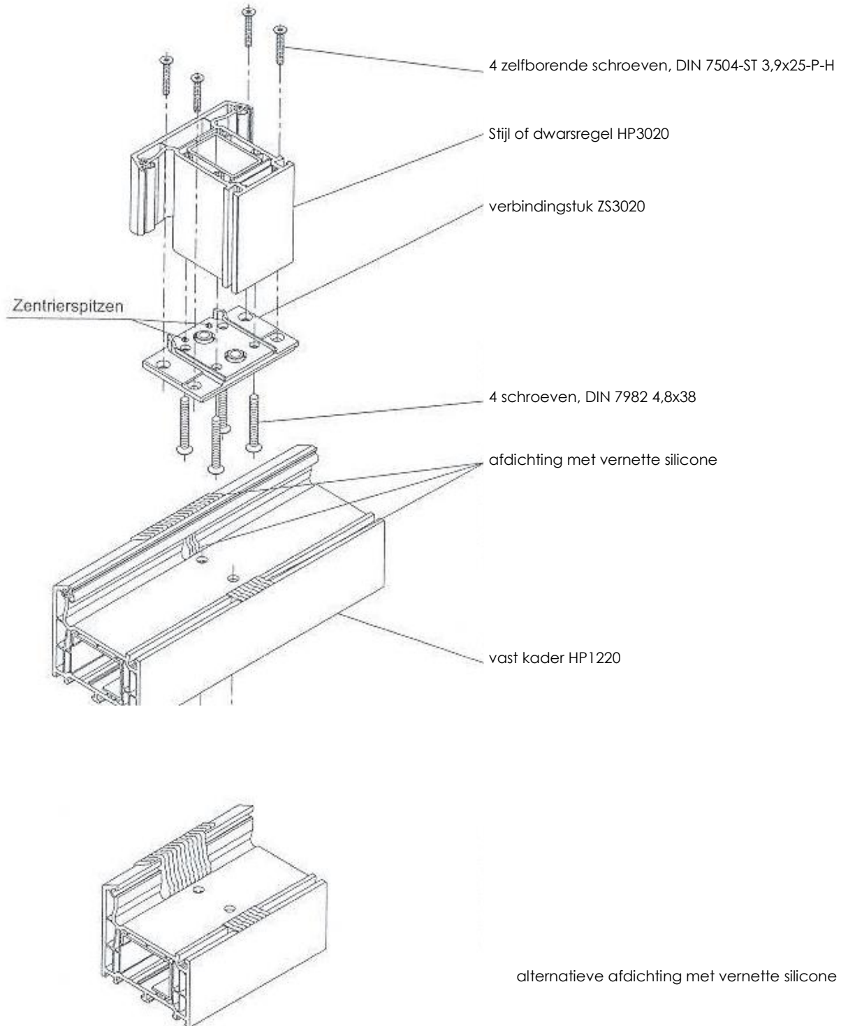
Figuur 6 – Mechanische T-verbinding
