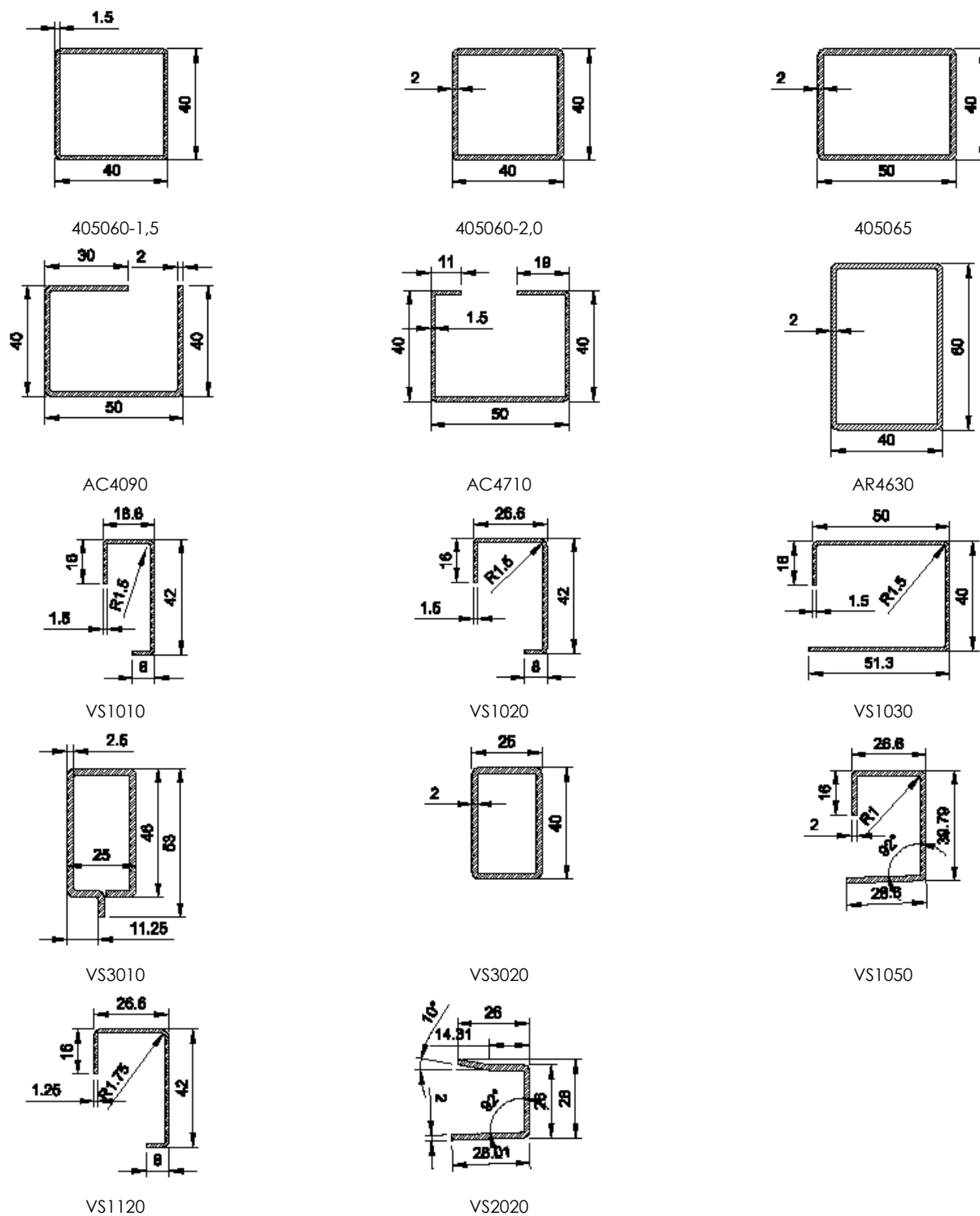
Figuur 4 – Versterkingsprofielen
