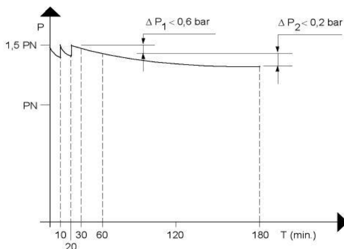
Fig. 1 – Contrôle d'étanchéité
